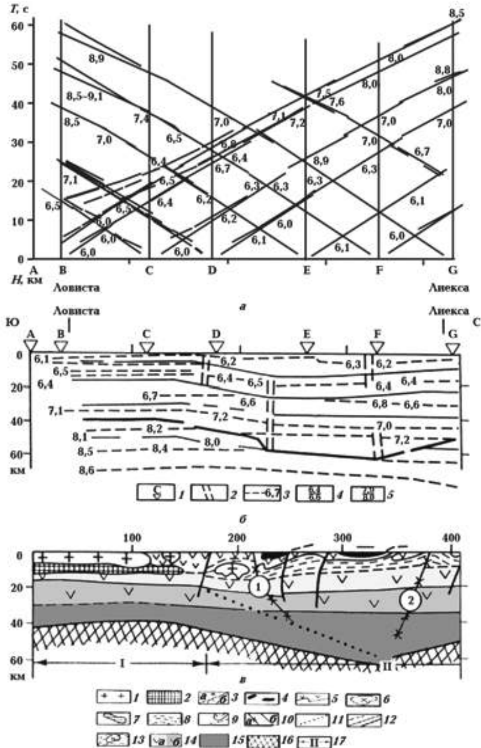
Рис. 2. Геолого-геофизический разрез земной коры по профилю Балтик [Luosto et al., 1990; Шаров, 1993; Mitrofanov et al., 1998]: a — системы наблюдаемых годографов; б — сейсмический разрез (1 — пункты взрыва; 2 — глубинные разломы; 3 — преломляющие границы с граничными скоростями, км/с; 4 — отражающие границы с характеристикой скорости, км/с; 5 — граница М, построенная по отраженным и преломленным волнам с характеристикой скорости, км/с); в — геолого-геофизическая модель (1 — рапакиви-граниты (1,7—1,6 млрд лет); 2 — габбро-анортозиты, диабазы (1,7—1,6 млрд лет); 3а — граниты и 3б — гранодиориты (1,9—1,8 млрд); 4 — перидотиты, серпентиниты, габброиды и основные вулканиты (2,0—1,9 млрд лет); 5 — вулканогенно-осадочные образования (2,2—1,8 млрд лет); 6 — граниты, гранодиориты (2,8—2,6 млрд лет); 7 — габброиды, габбро-анортозиты (2,6—2,8 млрд лет); 8 — архейские гнейсы и сланцы; 9 — геоэлектрические границы; 10а — главные и 10б — второстепенные разрывные нарушения; разломы (цифры в кружках): 1 — Колконярви, 2 — Сувавсяси; 11 — пологие границы, предполагаемые по геологическим данным; 12 — геофизические коровые границы; 13 — верхний слой (верхний этаж) ( V = 5,9 \pm 6,2 км/с, \sigma = 2,6 \pm 2,75 г/см 3 ); 14 — средний ( V = 6,3 \pm 6,5 км/с, \sigma = 2,75 \pm 2,9 г/см 3 ) и нижний ( V = 6,6 \pm 6,8 км/с, \sigma = 2,9 \pm 3,0 г/см 3 ); 15 — коромантийный слой ( V = 7,0 \pm 7,3 км/с, \sigma = 3,0 \pm 3,2 г/см 3 ); 16 — граница М, мантия ( V = 8,0 \pm 8,2 км/с, \sigma = 3,35 г/см 3 ); 17 — тектоническое районирование (I — Свекофеннский геоблок, II — Карельская кратон).
