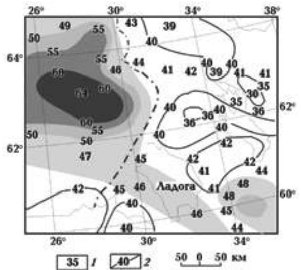
Рис. 7. Структурная схема раздела М юго-восточной части Фенноскандинавского щита: 1 — глубина (км) до раздела М по сейсмическим профилям, 2 — изогипсы раздела М, км.
