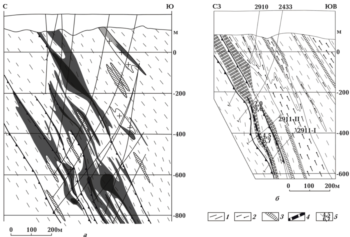
Рис. 5. Геологические разрезы Юрьевского уранового месторождения по профилю 92 (а) и Юрьевского рудопроявления золота по профилю 8 (б): 1 — биотитовые гнейсы; 2 — кордиеритовые гнейсы; 3 — аплит-пегматоидные граниты и пегматиты; 4 — золотосульфидные рудные тела; 5 — параметры золотых руд (в числителе — мощность, м; в знаменателе — содержание золота, г/т). Остальные условные обозначения см. на рис. 4.
