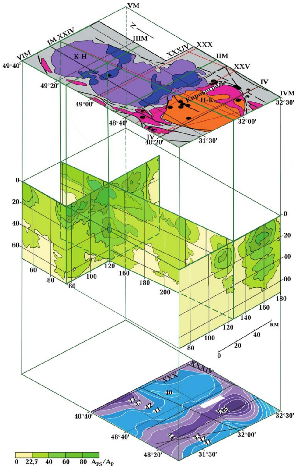
Рис. 11. Объемная сейсмогеологическая модель Кировоградского рудного района. Вверху — современный эрозионный срез рудного района, в средней части — каркасная блок-диаграмма поля обменных волн землетрясений, внизу — проекция месторождений урана, золота, лития на рельеф поверхности Мохо. Остальные пояснения в тексте.
