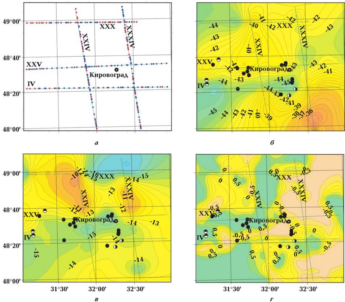
Рис. 10. Пространственные соотношения рельефа поверхностей М и К 2 и месторождений урана, золота, лития: а — расположение сейсмических профилей и точек определения глубины до поверхностей (красные отметки М, синие отметки К 2 ), б — схематическая карта рельефа М, в — схематическая карта рельефа К 2 , г — схема корреляции поверхностей М и К 2 . На схемах б, в, г показаны вертикальные проекции месторождений урана, золота, лития в соответствии с рис. 7.
