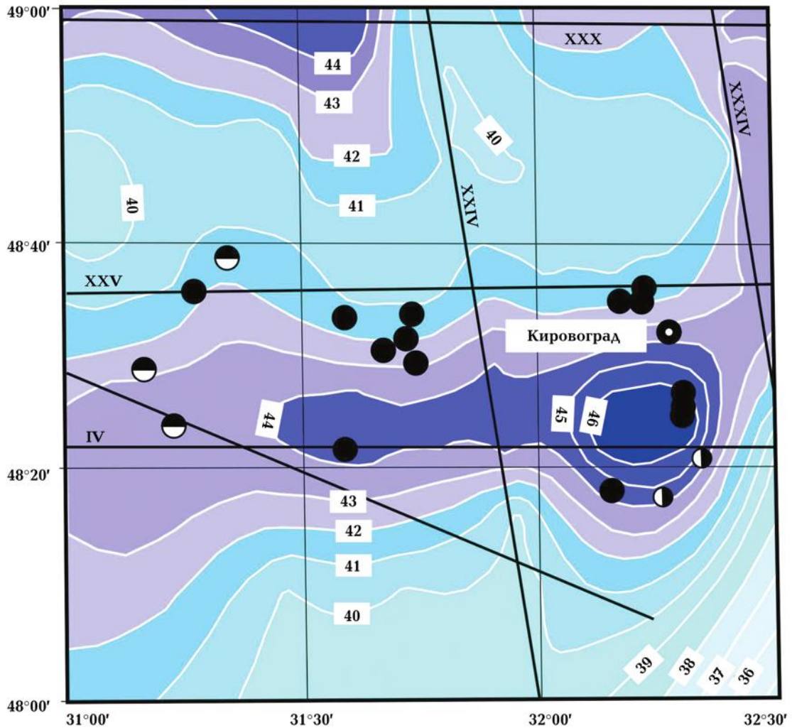
Рис. 9. Вертикальные проекции месторождений урана, золота, лития на рельеф раздела Мохо (отметки изолиний рельефа, км). Месторождения, профили ГСЗ и их номера нанесены согласно рис. 7.
