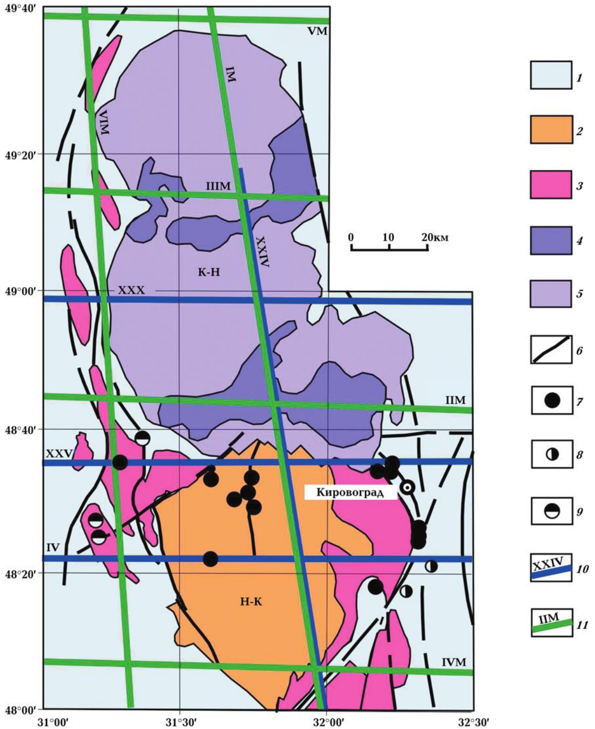
Рис. 7. Сейсмическая изученность Кировоградского рудного района: 1 — ингуло-ингулецька серия; 2, 3 — Новоукраїнсько-Кіровоградський масив (Н-К) (2 — диорит-монзонітова формація, 3 — граніт-мігматитова формація); 4, 5 — Корсунь-Новоміргородський масив (К-Н) (4 — габбро-анортозитова формація, 5 — рапаківі-гранітна формація); 6 — розломи; 7—9 — місця народження і рудопроявлення (7 — урана, 8 — золота, 9 — літія); 10 — профілі ГСЗ і їх номери; 11 — профілі МОВЗ і їх номери.
