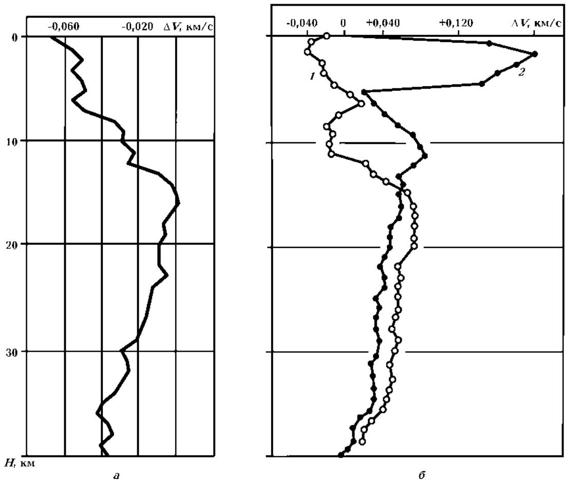
Рис. 8. Соотношения осредненных скоростей распространения продольных волн в коре Ингульского мегаблока ( V_{ин} ) и Украинского щита ( V_{уш} ), где \Delta V = V_{ин} - V_{уш} (а), и в вертикальном разрезе Новоукраинско-Кировоградского гранитоидного (1) и Корсунь-Новомиргородского рапакиви-анортозитового массивов (2) в сопоставлении со скоростью кривой Ингульского мегаблока, где \Delta V = 0 на тех же глубинах (б).
