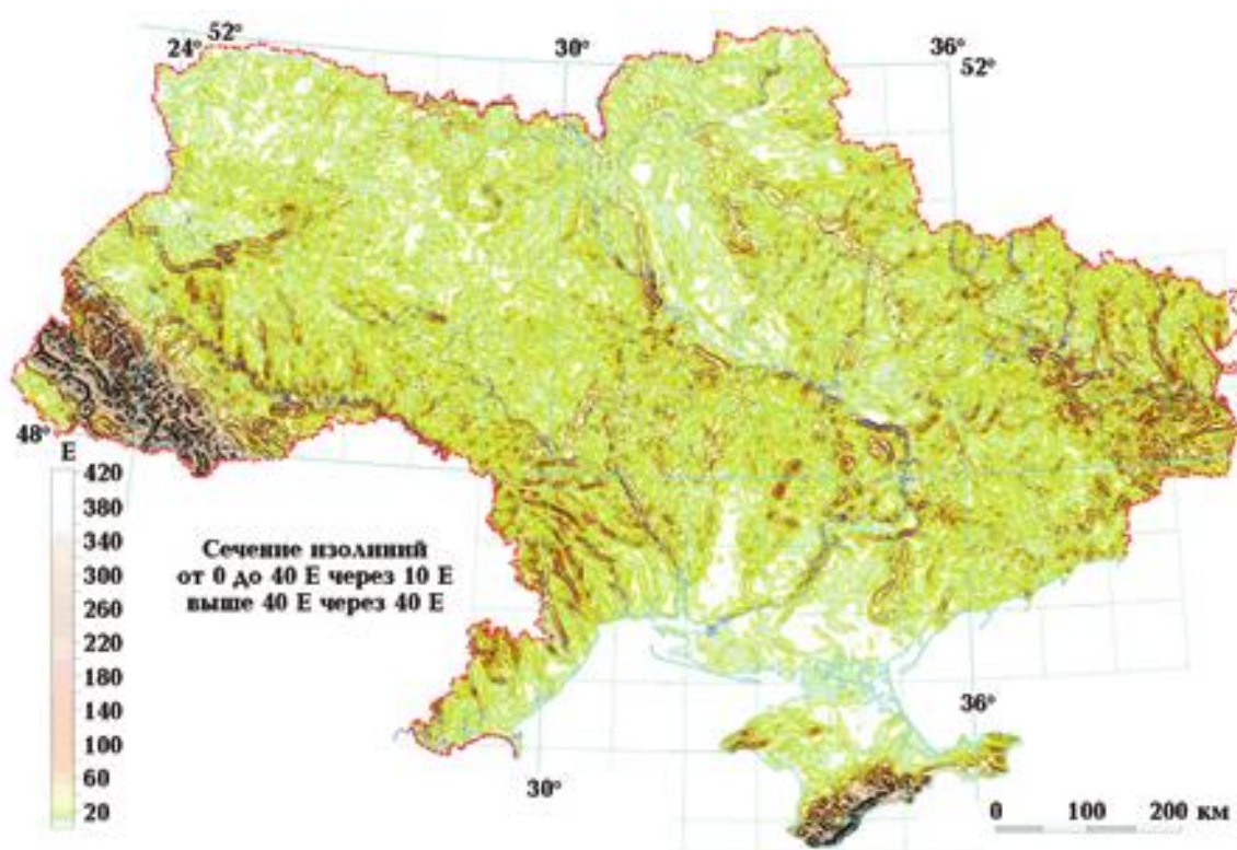
Рис. 4. Модуль полного горизонтального градиента поля силы тяжести для территории Украины.
