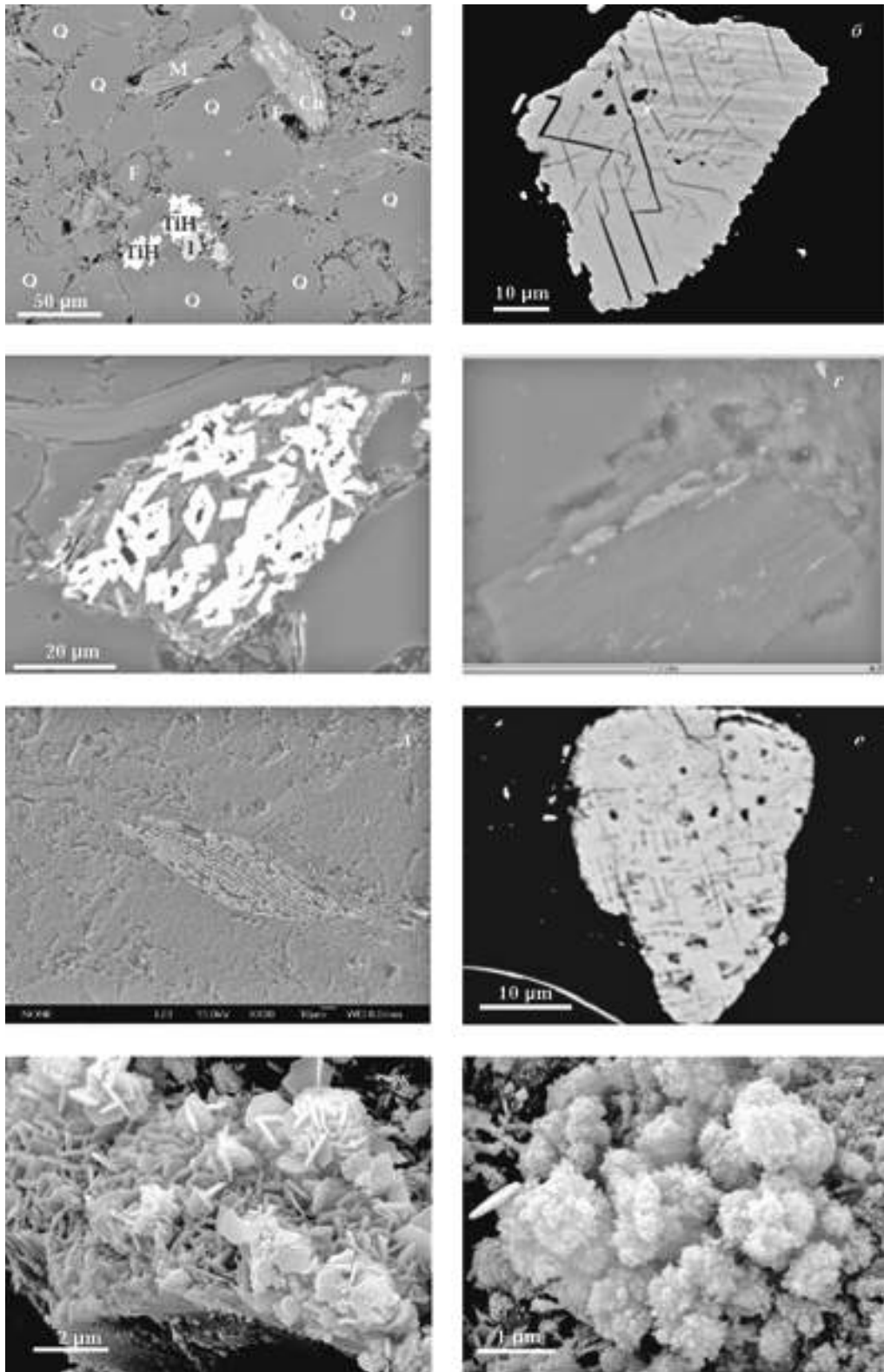
Рис. 11. Минералы железа — носители ЕОН в нижнедевонских красноцветах Подолии: a — BSE (back-scattered electron detector) изображение красноцветного песчаника; Q — кварц, F — полевоы шпат, M — мусковит, Ch — хлорит, TiH — титаногематит, I — ильменит; б — BSE — изображение детритового зерна первичного гематита с темными прослоями ильменита (тигрово-полосатое "tiger striped" ильменит-гематитовое прорастание); в—д — BSE — изображения кристаллов зеркального гематита в пост-биотит хлоритовых агрегатах; е — BSE — изображение зерна мартита; ж — SEM — изображение гексагональных зерен аутигенного гематита; з — SEM — изображение сращенных агрегатов зерен гематита типа "цветной капусты".
