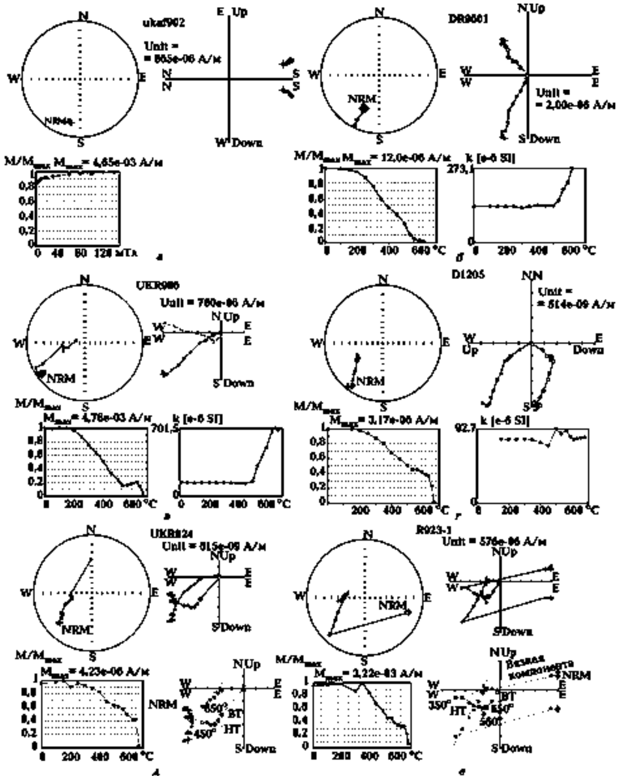
Рис. 3. Примеры ступенчатого размагничивания образцов красцветов Подольи переменным магнитным полем (а) и температурой, на которых выделяется только НТ-компонента (б), а также НТ- и ВТ-компоненты намагниченности (в—е). Приведены стереограммы (полюе / залитые круги — проекции векторов на верхнюю / нижнюю полусферу), нормированные кривые размагничивания ЕОН, изменение МВ при нагревах (б—г), диаграммы Зийдervельда (залитые / полые круги — проекции на горизонтальную / вертикальную плоскость) и примеры выделения на них компонент намагниченности (пунктирные линии на диаграммах (д, е)).
