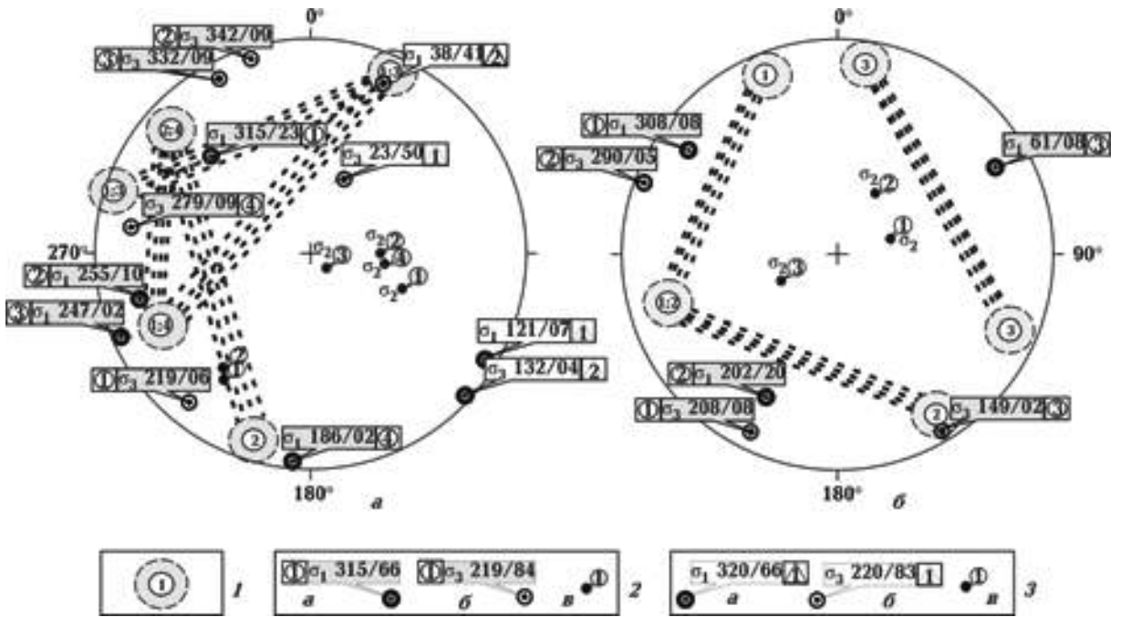
Рис. 6. Стереогаммы полюсов парагенетически связанных групп трещин Уманского (а) и Новоград-Волынского (б) массивов и оси главных нормальных напряжений по данным интерпретации парагенезисов трещин и зеркал скольжения: 1 — центры групп парагенетических связей трещин, 2 — парагенезисы трещин (а — \sigma_1 , б — \sigma_3 , в — \sigma_2 ), 3 — зеркала скольжения (а — \sigma_1 , б — \sigma_3 , в — \sigma_2 ).
