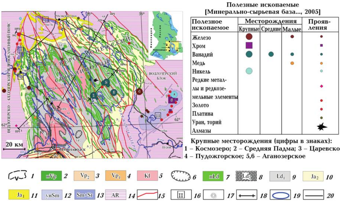
Рис. 1. Геологическая карта Северо-Онежского синклинория [Онежская..., 2011; Минерально-сырьевая..., 2005]. Неопротерозой: 1 — контуры вендских осадочных образований. Палеопротерозой. Вепсий (1,8—1,65 Ga); 2 — роупучейский комплекс. Габбродолериты, долериты, базальты, в т.ч. предполагаемые в акватории Онежского озера; 3 — шокшинский горизонт. Красноцветные кварцитопесчаники и кварциты, конгломераты; 4 — петрозаводский горизонт. Сероцветные песчаники, алевролиты, аргиллиты, конгломераты. Калевий (1,92—1,8 Ga); 5 — серо- и пестроцветные (иногда карбонат и углеродсодержащие) аргиллиты, алевролиты, кварцитопесчаники, конгломераты. Людиковий (2,1—1,92 Ga); 6 — наиболее интенсивная магнитная аномалия, вероятно, связанная с вулканическим центром людиковия; 7 — людиковийский и ятулийский магматические комплексы (нерасчлененные): перидотиты, габброиды, долериты, диориты и частично базальты; 8 — суйсарский горизонт. Пикриты, пикробазальты, базальты, туфы, туффимы и туфоконгломераты; 9 — заонежский горизонт. Шунгитоносные породы, аргеллиты, алевролиты, доломиты, базальты, андезитобазальты. Ятулий (2,3—2,1 Ga); 10 — онежский горизонт. Доломиты, гипсы, соли, ангидрит-магнетитовые породы, красноцветные алевролиты, базальты, долериты; 11 — сегозерский горизонт. Песчаники, кварцитопесчаники, аркозы, конгломераты, базальты, долериты. Сумий+Сариолий (2,5—2,3 Ga); 12 — бураковский комплекс. Дуниты, перидотиты, габбро-нориты, габбро, долериты, диориты; 13 — полимиктовые конгломераты, кварцитопесчаники, граувакки, базальты, андезитобазальты, туфы, туффиты. Архей (3,5—2,5 Ga); 14 — нерасчлененные метаморфиты по саамским и лолийским вулканогенным, магматогенным и осадочным образованиям; 15 — основные разломы; 16 — реликты (I — Кумсинский, II — Пальеозерский, III — Бураковский) сумийско-сариолийского рифтового пояса; 17 — Онежская параметрическая скважина (ОПС); 18 — фрагменты профилей МОВЗ (ПР1, ПР2, ПР6) и номера пикетов; 19 — контуры основных водоемов; 20 — основные дороги. Полезные ископаемые по Михайлову и др. [Минерально-сырьевая..., 2005].
