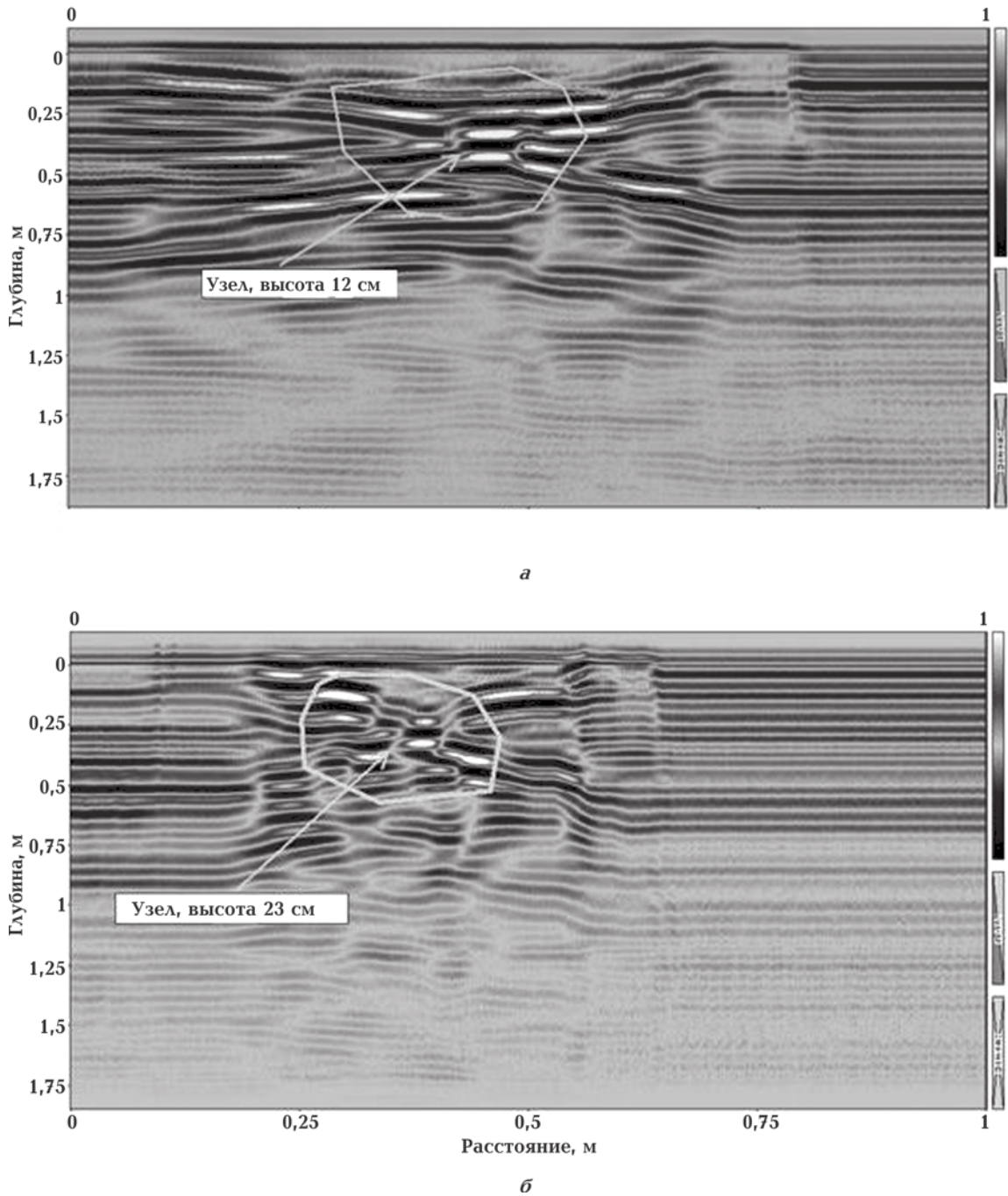
Рис. 5. Радарограмма для заполненной на 12 (а) и 23 (б) см водой полости.
