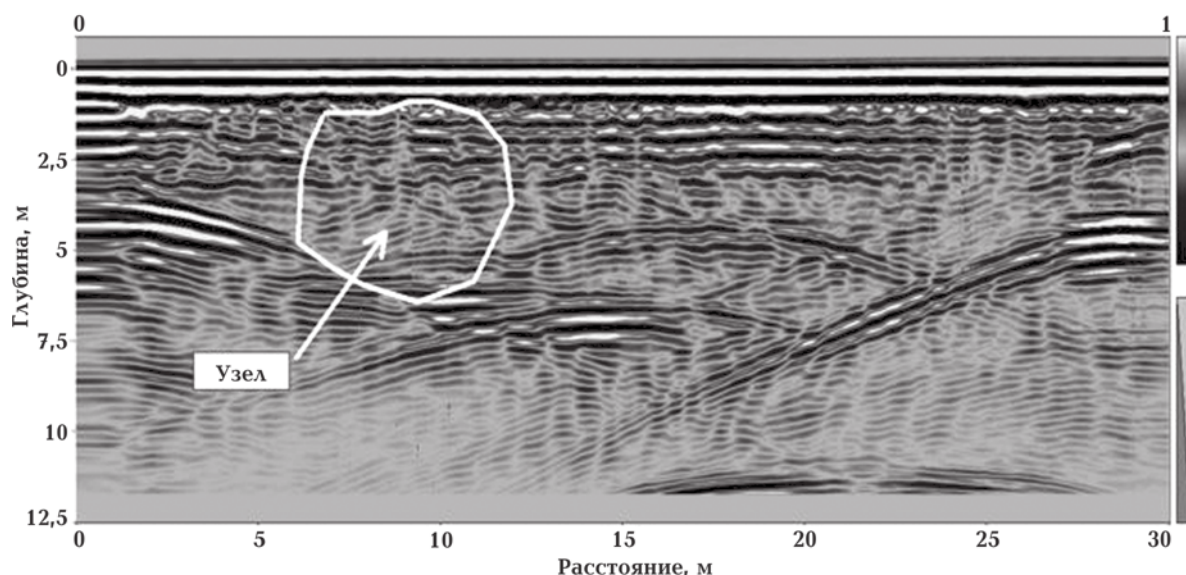
Рис. 7. Георадарный профиль в самом Кафедральном соборе Светицховели; стрелкой показано характерное для открытой полости «лучевое пересечение».
