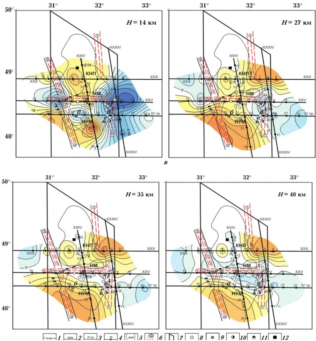
Рис. 2. Розташування Кіровоградського рудного району у тектонічних структурах центральної частини Українського щита. Ізолінії \Delta V : а — при H=0 км; б — при H=8 та H=9 км; в — при H=14 та H=27 км; г — при H=35 та H=40 км; 1 — ізолінії \Delta V , км/с; 2 — профіль ГСЗ; 3 — геотраверс IV; 4 — точки на профілях, де розраховано графіки V=f(H) (див. на рис. 1); 5 — контури геологічних структур (КНП — Корсунь-Новомиргородський плутон, НУМ — Новоукраїнський масив); 6 — зони розломів (цифри у кружках: 1 — Кіровоградська, 2 — Суботсько-Мошоринська, 3 — Звенигородсько-Братська); 7 — контур Кіровоградського рудного району; 8 — родовища урану; 9 — родовища урану, на яких наведено геологічні розрізи [Старостенко і др., 2010, 2011] (а — Ватутинське, б — Партизанське, в — Новокосятинівське, г — Северинське, д — Мічуринське, е — Юріївське); родовища та рудо прояви: 10 — золота, 11 — літію; 12 — титану.
