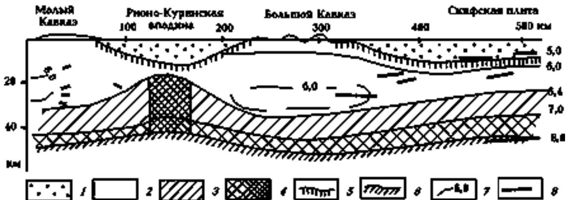
Рис. 7. Скоростная модель земной коры вдоль профиля ГСЗ Волгоград—Нахичевань, по данным [Pavlenkova, 1996]: 1 — осадочный чехол; 2—4 — слои консолидированной коры со скоростями P -волн (2 — 6,0 \div 6,4 км/с, 3 — 6,5 \div 6,7 км/с, 4 — 6,8 \div 7,2 км/с); 5 — поверхность фундамента; 6 — граница М; 7 — отражающие площадки; 8 — изолинии скорости, км/с.
