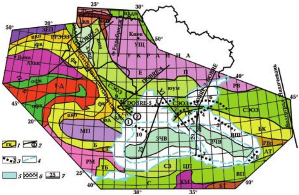
Рис. 1. Схема основных тектонических структур исследуемого региона. Компиляция материалов и карт, по [Тектонічна ..., 2007; Okay, Tüysüz, 1999; Юдин, 2007; Афанасенков и др., 2007; Hippolite, 2002; Koperding et al., 2010; Csontos, Vörös, 2004]. Составили Гинтов О.Б., Муровская А.В.: 1 — контуры основных тектонических структур и их обозначения, 2 — разломы и их номера (1 — Печенега-Камена, 2 — Кагульский), 3 — прогибы и их номера (1 — Каркинитский, 2 — Предгорнокрымский, 3 — Сорокина, 4 — Керченско-Таманский, 5 — Туапсинский, 6 — Индоло-Кубанский, 7 — Синопский, 8 — Гурийский, 9 — Преддобруджинский, 10 — Истринский), 4 — глубоководные впадины, 5 — океаническая и субокеаническая кора, 6 — Трансевропейская шовная зона, 7 — геотраверсы и профили ГСЗ. Тектонические структуры: Альк — Алькапа, АТ — Аджаро-Триалетия, Б — Балканиды, БК — Большой Кавказ, ВЕП — Восточно-Европейская платформа, ВП — Восточные Понтиды, ВПМ — Вольно-Подольская моноклиналь, ВПП — Вольно-Полесский прогиб, ВЧВ — Восточно-Черноморская впадина, ВШ — Вал Шатского, ЗЕП — Западно-Европейская платформа, ЗЧВ — Западно-Черноморская впадина, КВ — Ковельский выступ, КМ — Киршехирский массив, ЛЛПП — Львовско-Люблинский палеозойский прогиб, МП — Мизийская платформа, ОФК — площади широкого распространения офиолитовых комплексов (Вардар, Мелиата и др.), ПБ — Паннонский бассейн, ПДДВ — Припятско-Днепровско-Донецкая впадина, ПКП — Предкарпатский прогиб, ПС — Полесская седловина, РВ — Ростовский выступ, РВп — Рионская впадина, РМ — Родопский массив, РРЭОЗ — Рава-Русская эпиорогенная зона, С — Сакарция, СГ — Среднегорье, СД — Северная Добруджа, СЗ — Стамбульская зона, СУГЗ — Северо-Украинская горстовая зона, СЭОЗ — Скифская эпиорогенная зона, ТБ — Тракийский бассейн, Т-Д — Тиссия-Дакия, УЩ — Украинский щит, ФК — Флишевые Карпаты, ЦД — Центральная Добруджа, ЦП — Центральные Понтиды, ЮД — Южная Добруджа, ЮУМ — Южно-Украинская моноклиналь.
