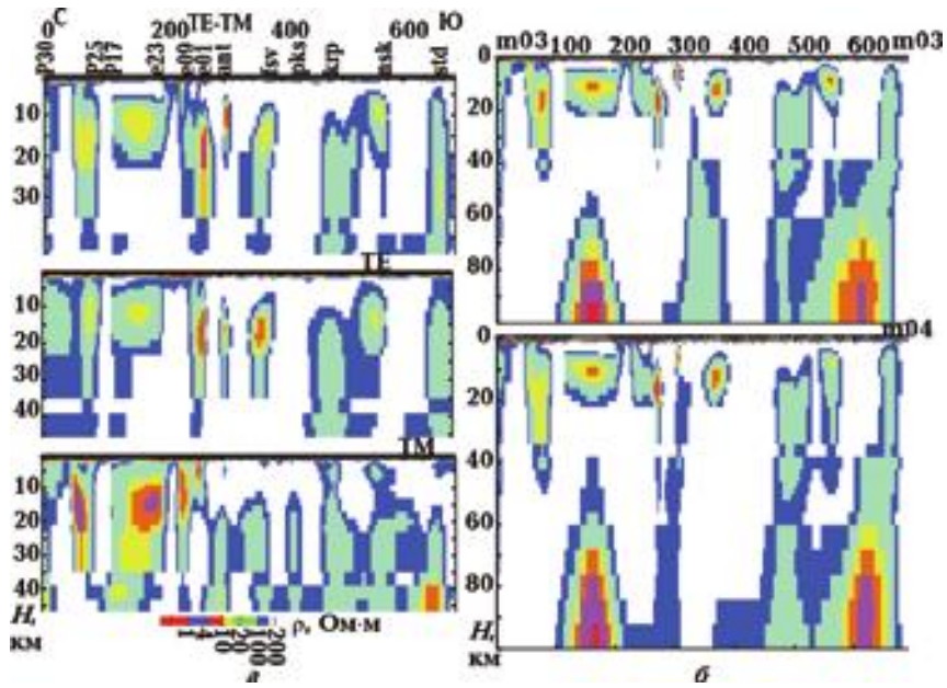
Рис. 3. Геоэлектрические модели, полученные с использованием различных мод: а — вариант I, б — вариант II.
