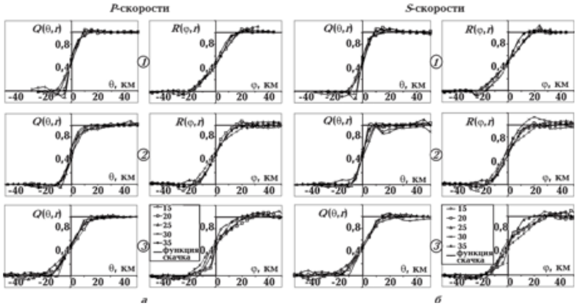
Рис. 6. Функции Q(\theta, r) и R(\varphi, r) [Гобаренко. Яновская, 1983], определяющие интервалы сглаживания по горизонтальным координатам \theta, \varphi для P -волн (а) и S -волн (б) для трех разных точек (точки 1, 2 и 3 на рис. 4) района исследований. Вектор r соответствует координатам заданной точки.
