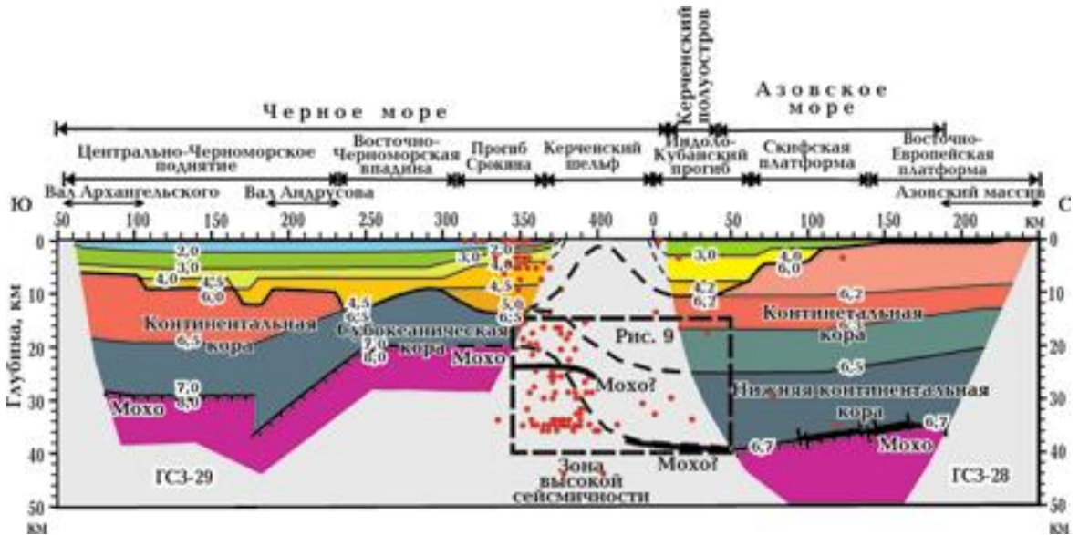
Рис. 11. Вертикальный разрез сейсотомографической модели (см. рис. 9 в пунктирном прямоугольнике), объединенный со скоростным разрезом по профилю 28—29 в интерпретации [Yegorova et al., 2010]. Кружками показаны спроецированные на профиль очаги землетрясений в пределах 20-километровой области к западу и востоку от профиля. Тонким черным пунктиром в области отсутствия скоростной модели по профилю 28—29 показана интерполяция скоростной модели, а утолщенная черная линия соответствует пунктирной линии, оконтуренной по данным соотношения V_p/V_s томографической модели на рис. 8 (Мохо?).
