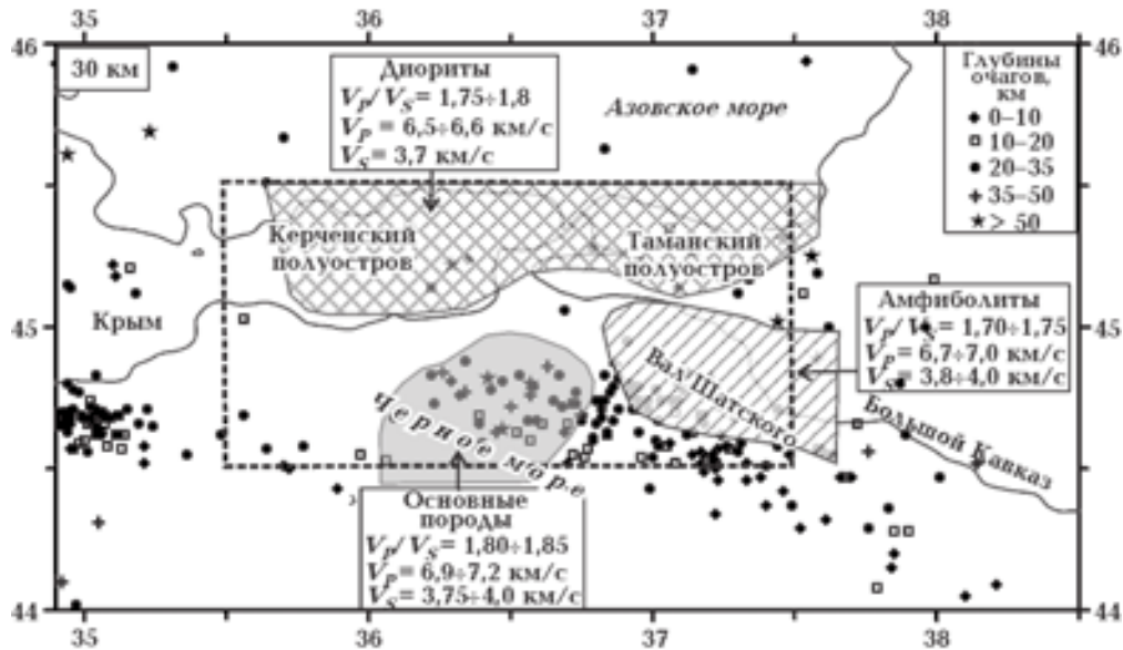
Рис. 12. Петрологическая интерпретация основных аномальных зон. Показана на примере глубинного среза ( H=30 км) локальной сейсмографической модели района исследований (оконтурен пунктиром) и на фоне слабой ( m_b \leq 3 ) сейсмичности региона.
