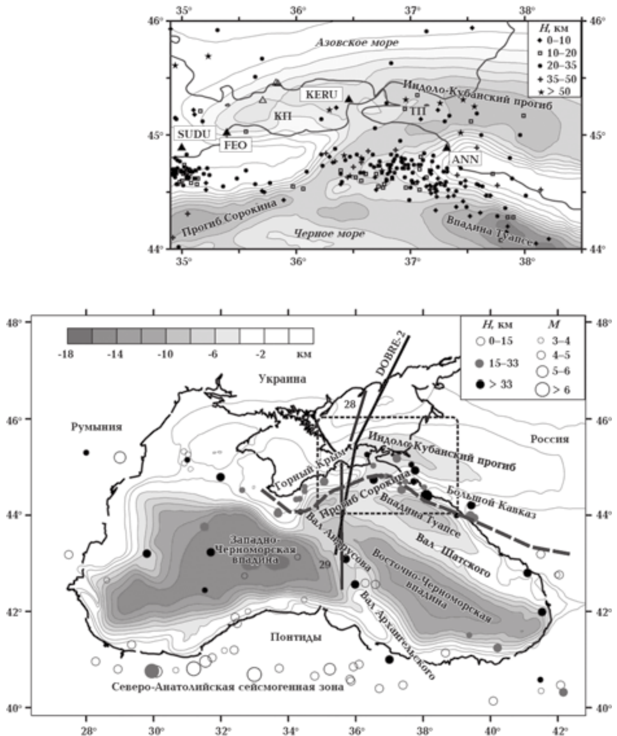
Рис. 1. Основные тектонические элементы района исследований (окоптурен пунктиром) и сейсмичность Черноморского региона [Yegorova, Gobaigenko, 2010] на фоне структурной карты кровли меловых отложений.
