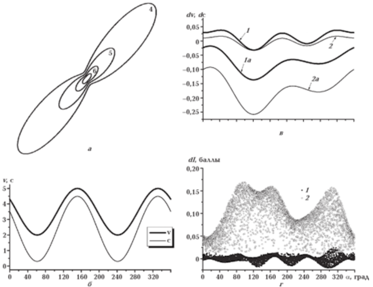
Рис. 2. Тестируемый пример заданного модельного анизотропного макросейсмического поля: a — изосейсты теоретического макросейсмического поля; b — заданные функции v_0(\alpha) , c_0(\alpha) ; v — отклонения dv(\alpha) : 1 — без помех, 1a — с помехой \pm 1 балл; отклонения dc(\alpha) : 2 — без помех, 2a — с помехой \pm 1 балл; г — отклонения расчетных интенсивностей относительно заданных: 1 — без помех, 2 — с помехой \pm 1 балл.
