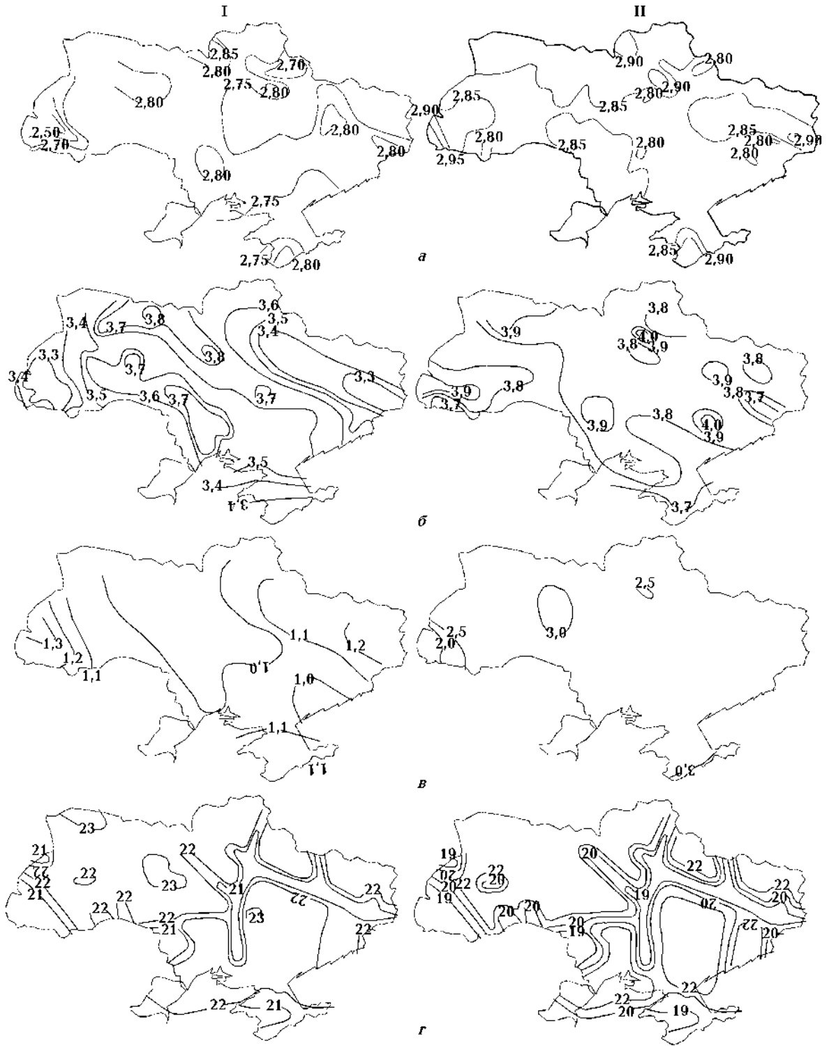
Рис. 4. Распределение на глубине 7,5 (I) и 22,5 (II) км плотности пород, \text{г/см}^3 (а), скорости распространения поперечных сейсмических волн, \text{км/с} (б), удельной упругой энергоемкости, 10^6 \text{ Дж/м}^3 (в) и вязкости (изолинии — показатель степени — 10^9 \text{ Па} \cdot \text{с} ) (г) для территории Украины.
