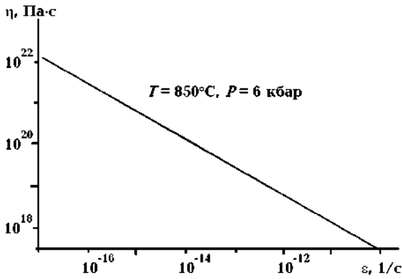
Рис. 5. Зависимость вязкости диабаза от скорости деформации [Геря, 1999].
