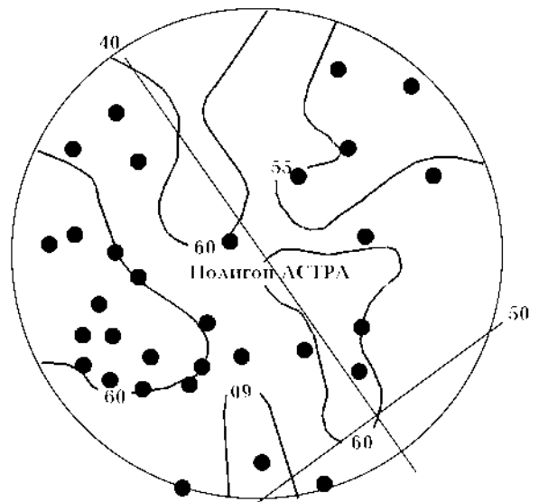
Рис. 3. Распределение K ( \text{г} \cdot \text{см}^{-3} \cdot \text{км}^2 \cdot \text{с}^{-2} ) в слое с глубинами кровли и подошвы 6 и 9 км (изолинии), по [Геотраверс ..., 2002], на полигоне АСТРА и эпицентры землетрясений (точки) [Геотраверс ..., 2002; Надежка и др., 2008; Савко и др., 2008].
