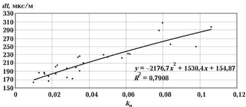
Рис. 6. Кореляційна залежність між коефіцієнтом пористості ( k_{\text{п}} ) та інтервальним часом ( dt ).
