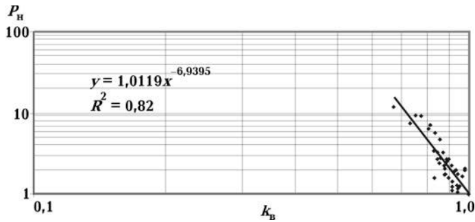
Рис. 4. Кореляційна залежність між коефіцієнтом водонасиченості ( k_B ) та коефіцієнтом збільшення опору ( P_H ) для алеволітів: P_H = 1,012 k_B^{-6,94} при R^2 = 0,82 .
