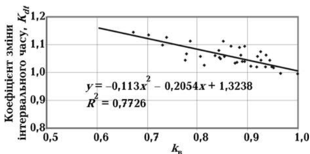
Рис. 8. Кореляційна залежність між коефіцієнтом водонасиченості ( k_{\text{в}} ) та коефіцієнтом зміни інтервального часу ( K_{dt} ) для алевролітів: K_{dt} = -0,113 k_{\text{в}}^2 - 0,205 k_{\text{в}} + 1,324 при R^2 = 0,773 .
