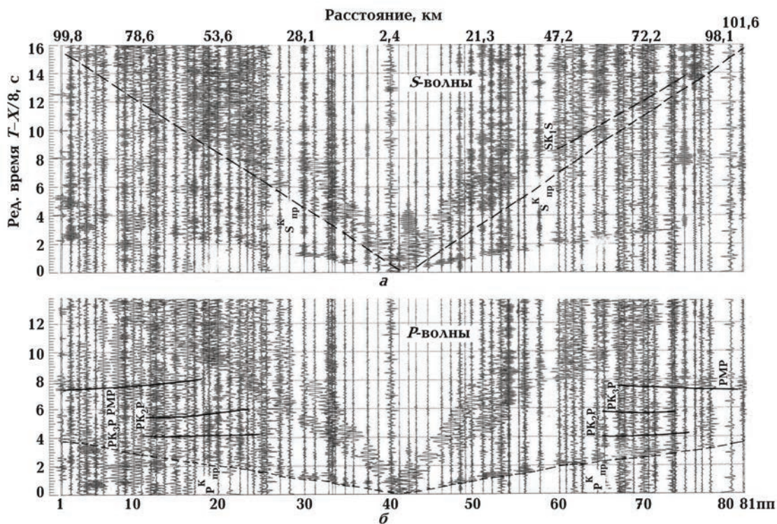
Рис. 5. Монтажи сейсмограмм ПВ 41 ( V_P = 8,0 км/с) Z-компоненты (а) X-компоненты (б).
