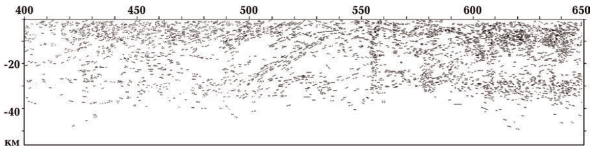
Рис. 2. Схематизированный разрез МОГТ земной коры участка Кандалакша — Кемь геотранверса 1-ЕВ [Сейсмогеологическая ..., 1998].
