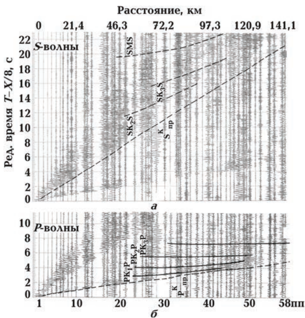
Рис. 4. Монтажи сейсмограмм ПВ 1 ( V_P = 8,0 км/с) Z-компоненты (а), X-компоненты (б).
