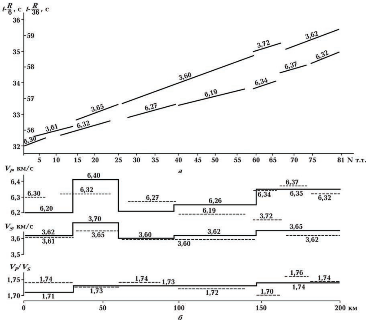
Рис. 6. Изменения V_P , V_S и V_P/V_S по профилю Кандалакша — Кемь.
