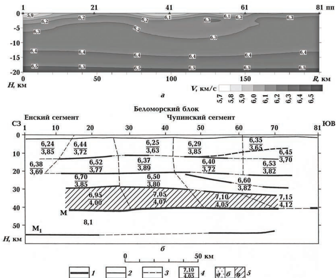
Рис. 7. Сейсмотомографический разрез (а) по профилю Кандалакша — Кемь. Глубинный сейсмический разрез ГСЗ—МОВЗ (б): 1—3 — границы (1 — построенные по нескольким типам волн, 2 — по одному типу волн, 3 — теоретические, соответствующие решению прямой задачи), 4 — скорости P - и S -волн, 5 — содержание \text{SiO}_2 , вес. проценты (а — более 66; б — 56—65; в — менее 55).
