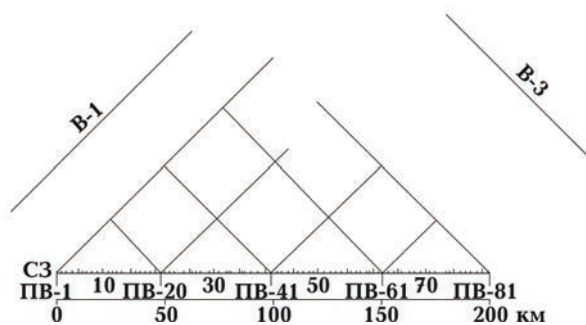
Рис. 3. Система наблюдений по геотраверсу 1-ЕВ (участок Кандавакша — Кемь).
