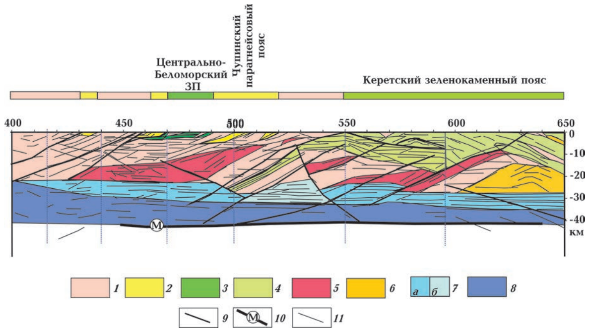
Рис. 8. Геолого-геофизический разрез земной коры по профилю Кандалакша — Кемь: 1—5 — позднеархейские (1 — гранитогнейсы (преимущественно ТТГ)), 2 — парагнейсы Чупинского пояса, 3 — амфиболиты и ультрамафиты (офиолиты), 4 — зеленокаменный комплекс, 5 — гранулит-эндербит-чарнокитовый комплекс); 6 — раннепротерозойские гранулиты (чарнокиты); 7 — нижнекоровые образования с многочисленными горизонтальными отражающими поверхностями (относительно высокоскоростные (а), относительно низкоскоростные (б)); 8 — нижнекоровые породы; 9 — разломы; 10 — граница Мохо; 11 — сейсмоотражающие поверхности.
