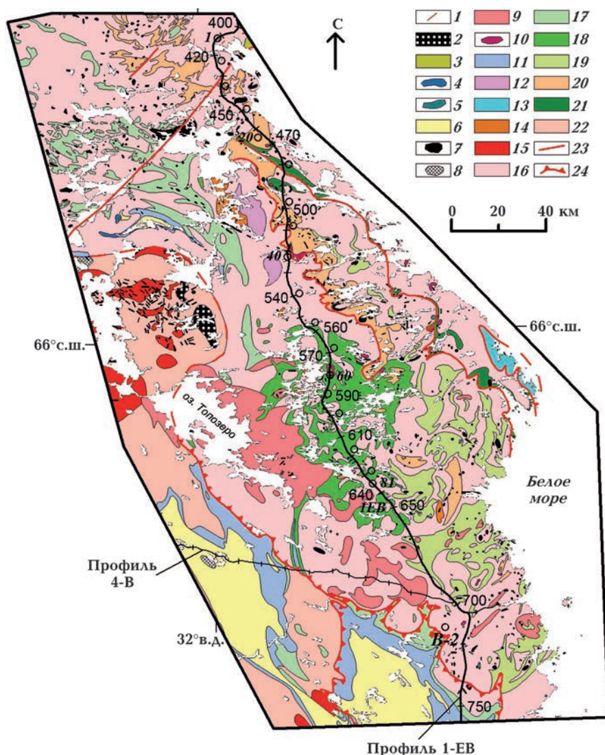
Рис. 1. Схема геологического строения [Слабунов, 2008] и расположение сейсмических профилей МОГТ 1-ЕВ и 4В, ГСЗ источников и приемников (круги) на северо-востоке Карелии: 1 — палеозойские дайки щелочных пород; 2—8 — палеопротерозойские образования (2 — щелочной Тикшозерско-Елетьозерский комплекс (1745—1827 млн лет), 3 — Колвицкий метаморфический комплекс, 4 — мафит-ультрамафитовый комплекс (Каменноозерский), 5 — комплекс коронитовых (гранатовых) габбро (2115 млн лет), 6 — ятулийские (2,3—2,0 млрд лет) вулканогенные и осадочные комплексы, 7 — дайки габброноритов (Карельская провинция) и комплекс лерцолитов-габброноритов БПП (2440—2390 млн лет), 8 — комплекс расслоенных интрузий (2450—2440 млн лет)); 9 — метачарнокиты топоверского типа; 10 — комплекс габброанортозитов (2,45—2,40 млрд лет); 11 — сумийские, сариолийские (2,5—2,3 млрд лет) вулканогенные и осадочные комплексы; 12—15 — неоархейские комплексы (12 — чарнокиты Нотозерского ГЭЧ комплекса (2756 млн лет), 13 — Гридинский эклогитсодержащий комплекс, 14 — эндербиты Нотозерского ГЭЧ комплекса (2778 млн лет), 15 — санукитоиды (2724 млн лет)); 16 — гранитоиды БПП (2,81—2,7 млрд лет); 17 — неоархейские (2778—2750 млн лет) зеленокаменные комплексы; 18—21 — мезоархейские супракrustальные комплексы (18 — Керетьозерский зеленокаменный, 19 — глубокометаморфизованные зеленокаменные (нерасчлененные), 20 — парагнейсы Чупинского пояса, 21 — офиолитоиды Центрально-Беломорского ЗКП); 22 — гранитоиды Карельского неоархейского кратона (3,5—2,65 млрд лет); 23 — предполагаемые разломы; 24 — палеопротерозойские надвиги.
