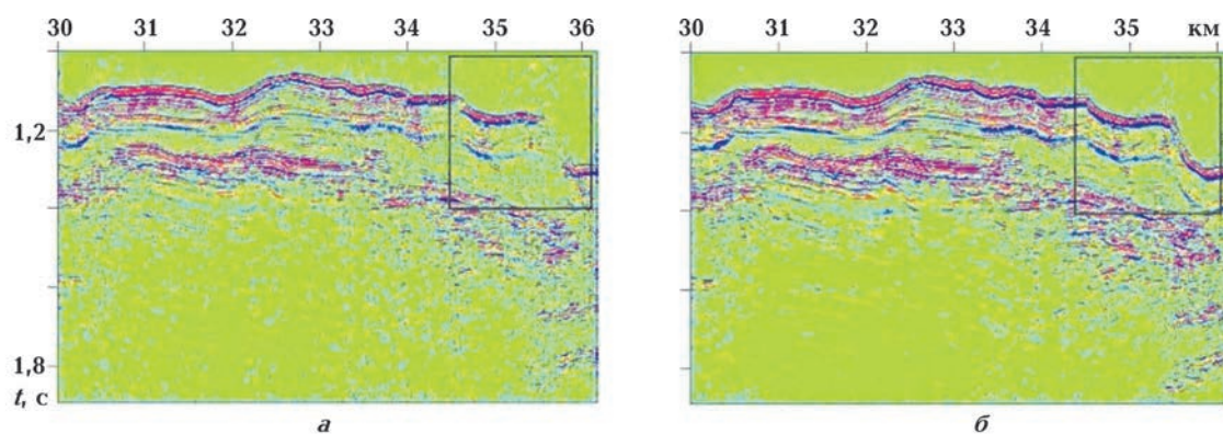
Рис. 6. Фрагменты временного разреза в интервале 34 000—36 000 м: а — сумма ОГТ; б — результат применения конечно-разностной полноволновой миграции суммы ОГТ во временном масштабе глубин. Прямоугольником выделен участок с нарушениями, где показана эффективность применения миграции.
