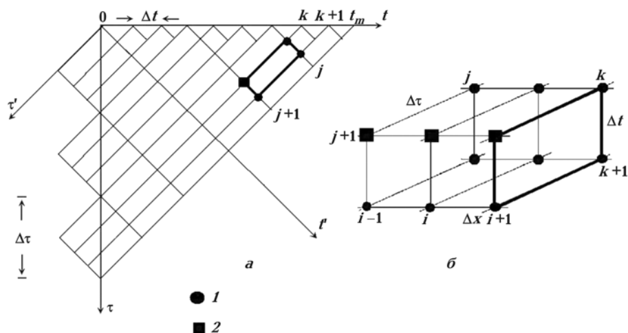
Рис. 4. Прямоугольная сетка обратного полноволнового продолжения поля: a — сечение сетки в плоскости; б — трехмерный 12-точечный шаблон (1 — узлы сетки, в которых волновое поле определено, 2 — узлы сетки, в которых волновое поле определяется).
