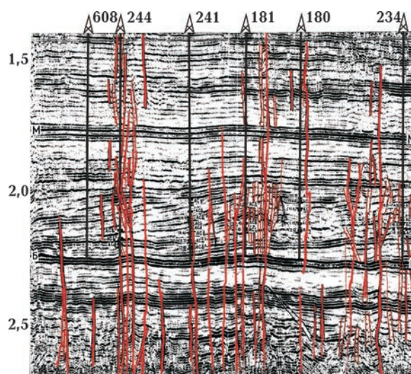
Рис. 2. Сейсмический временной разрез на Приобском месторождении.
