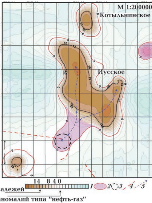
Рис. 11. Карта аномальных зон типа “залежь углеводородов” в районе Полутынской площади, Иусского и Котлынинского месторождений УВ (Шамимский нефтегазоносный район, Россия): 1 — шкала интенсивности аномального отклика (в единицах среднего пластового давления (МПа)); 2 — зона аномалий типа “газ”; 3 — положение Иусского объекта (геосолитона); 4 — тектонические нарушения; 5 — возможные пути миграции флюидов.
