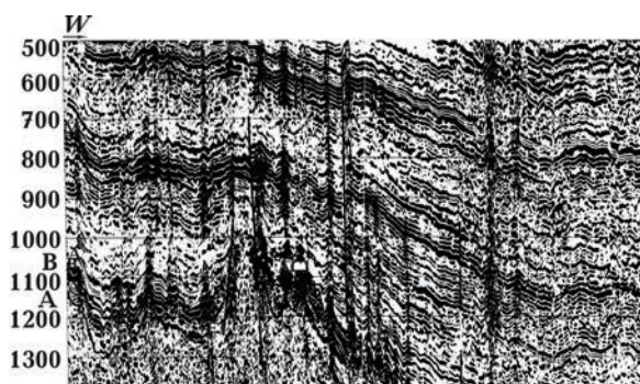
Рис. 1. Временной сейсмический разрез в районе сочленения Урала и Западной Сибири. Четко прослеживаются неотектонические трубки, проникающие от фундамента через юрские, меловые и третичные отложения до земной поверхности.
