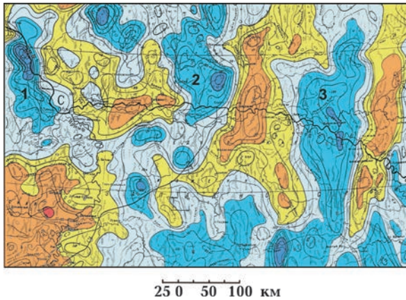
Рис. 8. Карта гравитационного поля в районе Краснolenинского (1), Сургутского (2) и Нижневартoвского (3) сводов. Отрицательные значения — в синих тонах, положительные — в красных.
