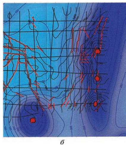
Рис. 5. Карты гравитационного (а) и магнитного (б) полей.
