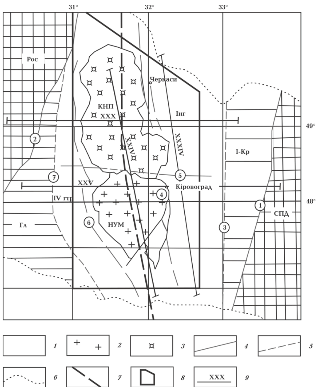
Рис. 1. Розташування Кіровоградського рудного району у тектонічних структурах центральної частини Українського щита: 1 — інгуло-інгулецька серія; 2 — гранітоїди; 3 — рапаківи, анортозити; зони розломів (цифри у кружечках): 4 — міжблокові (1 — Криворізько-Кременчуцька, 2 — Тальнівська); 5 — внутрішньоблокові (3 — Західноінгулецька, 4 — Кіровоградська, 5 — Суботсько-Мошоринська, 6 — Звенигородсько-Братська, 7 — Первомайська); 6 — контур Українського щита; 7 — трансрегіональний тектонічний шов Херсон—Смоленськ; 8 — контур Кіровоградського рудного району (КРР); 9 — профілі ГСЗ; мегаблоки: Інг — Інгулецький, Рос — Росинсько-Тікицький, СПД — Середньопридніпровський; шовні зони: Гл — Голованівська, І-Кр — Інгулецько-Криворізька; КНП — Корсунь-Новомиргородський плутон, НУМ — Новоукраїнський масив.
