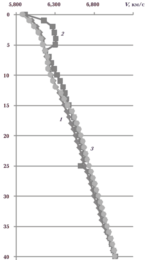
Рис. 6. Осереднені графіки \Delta V=f(H) : 1 — Кіровоградського рудного району (КРР); 2 — Корсунь-Новомиргородського плутону (КНП); 3 — Новоукраїнського масиву (НУМ).
