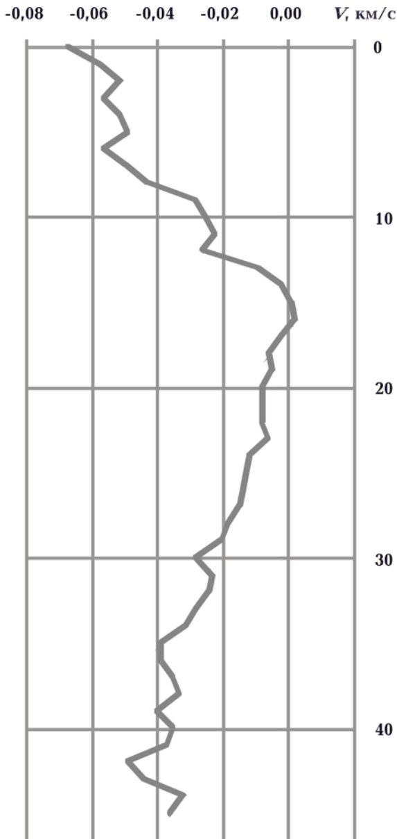
Рис. 3. Різниця \Delta V = V_{\text{ЦІБ}} - V_{\text{УЦ}} між осередненими сейсмічними швидкостями у земній корі центральної частини Інгульського мегаблока ( V_{\text{ЦІБ}} ) та Українського щита ( V_{\text{УЦ}} ).
