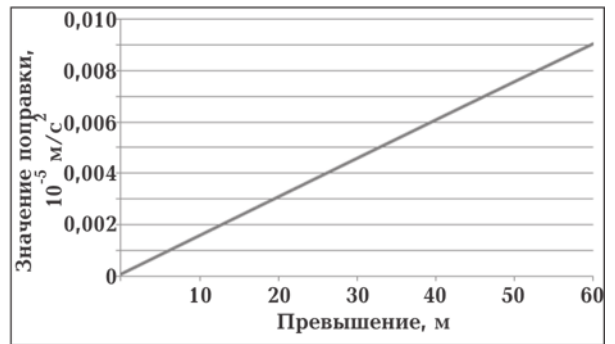
Рис. 6. Поправка (а) и погрешность в поправке (б) за влияние рельефа для средней зоны.
