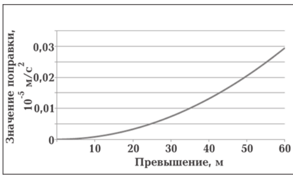
Рис. 8. Поправка (а) и погрешность в поправке (б) за влияние рельефа для дальней зоны № 2.
