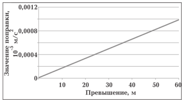
Рис. 8. Поправка (а) и погрешность в поправке (б) за влияние рельефа для дальней зоны № 2.
