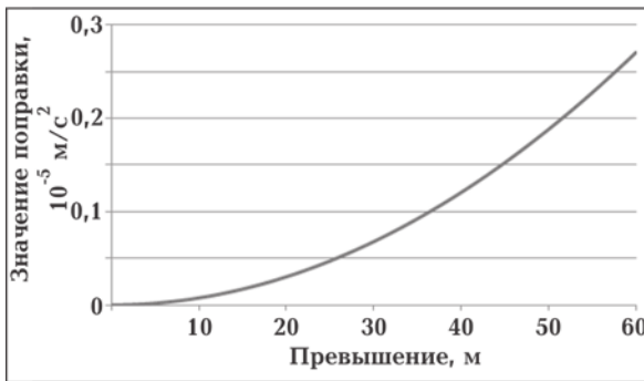
Рис. 6. Поправка (а) и погрешность в поправке (б) за влияние рельефа для средней зоны.
