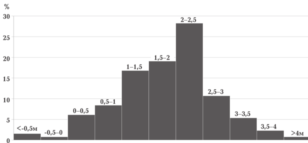
Рис. 4. Гистограмма отклонения между высотами по данным НППС и SRTM в точках НППС.
