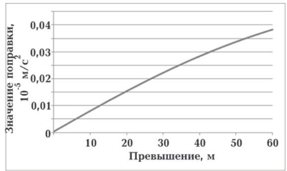
Рис. 6. Поправка (а) и погрешность в поправке (б) за влияние рельефа для средней зоны.
