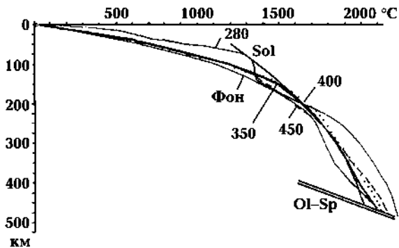
Рис. 4. Расчетная тепловая модель палеозойской геосинклинали Карпат. Условные обозначения см. на рис. 2.
