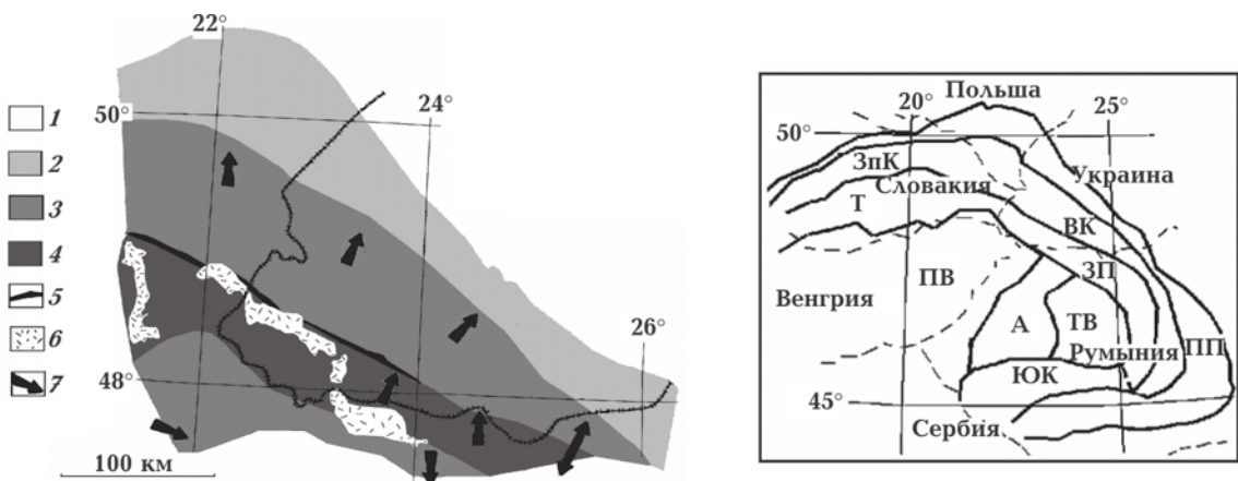
Рис. 1. Размещение геосинклиналиальных зон Восточных Карпат на территории Украины и в ближайших окрестностях: 1 — северо-восточный платформенный форланд Карпатской геосинклинали, 2 — Предкарпатский прогиб, 3 — зоны Складчатых Карпат и Дебреценская, 4 — зона Закарпатских прогибов, 5 — зона Пьенинских утесов, 6 — молодые вулканиты, 7 — направление надвигов. На врезке — тектонические единицы Карпат и границы государств: ПП — Предкарпатский прогиб, ЗпК — Западные Карпаты, ТК — Татры, ПВ — Паннонская впадина, ЗП — Закарпатские прогибы, А — Апусени, ТВ — Трансильванская впадина, ЮК — Южные Карпаты, Украина, Венгрия, Румыния, Сербия.
