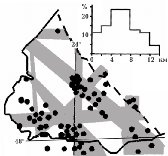
Рис. 15. Эпицентры землетрясений Украинских Карпат (черные точки) [Атлас..., 2002; Сафронов, 2005], зоны разломов, активных в последние 3 млн лет (серые полосы) [Верховцев, 2006], и гистограмма распределения глубин гипоцентров [Сафронов, 2005; Назаревич, 2005].
