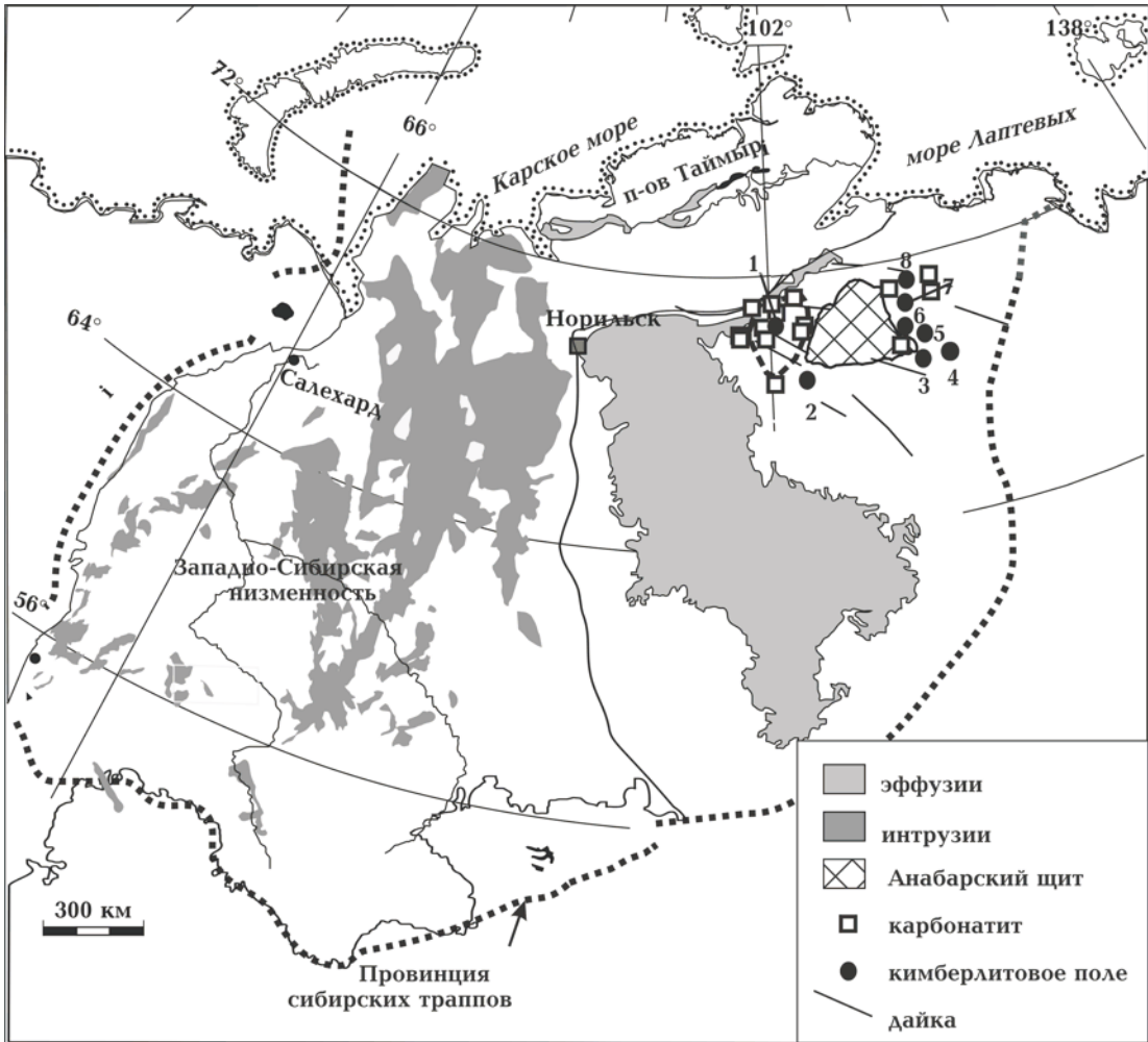
Рис. 2. Сибирские траппы (251—249 млн лет; светлосерое (эффузии) и темносерое (интрузии) поля), карбонатиты Маймечо-Котуйской и Анабарской провинций щелочного магматизма (250 млн лет; квадраты) и нижнетриассовые кимберлитовые поля Оленек-Анабарской зоны и Красноярского края (кружки: 1 — Котуйское, 2 — Харамайское, 3 — Куранахское, 4 — Лучаканское, 5 — Дюкенское, 6 — Ары-Мастахское, 7 — Старореченское, 8 — Орто-Ыаргынское).
