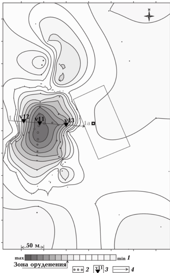
Рис. 4. Локальная аномалия типа «зона уранового оруденения» на площади работ: 1 — шкала интенсивности аномалий; 2 — отдельные пункты съемки СКИП; 3 — пункт ВЭРЗ; 4 — линия разреза.
