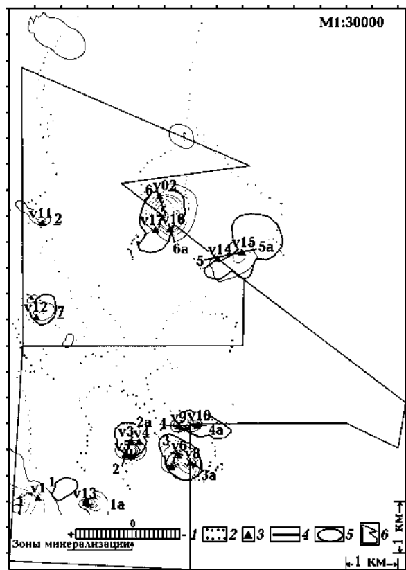
Рис. 6. Карта геоэлектрических аномалий типа «зона золоторудного оруденения» на участке «АР» (по данным съемки СКИП): 1 — шкала интенсивности поля СКИП; 2 — точки съемки СКИП; 3 — пункты ВЭРЗ; 4 — положение профилей №№ 1—6 по данным ВЭРЗ; 5 — зоны золоторудного оруденения по спутниковым данным; 6 — контуры участка работ.
