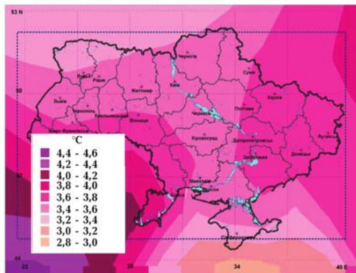
Рис. 5. Зміна в Україні річних температур повітря (а) і кількості опадів, % (б), середніх за десятиріччя XXI ст., порівняно з періодом 2001—2010 рр. Дані ансамблю 4 розрахунків моделі ECHAM5/MPI-OM за сценарієм А1В.
