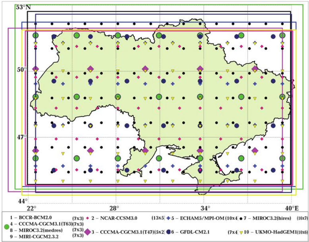
Рис. 1. Розрахункові сітки МЗЦАО за даними табл. 1 і відповідні їм області прогнозування клімату (рамки) для території України.
