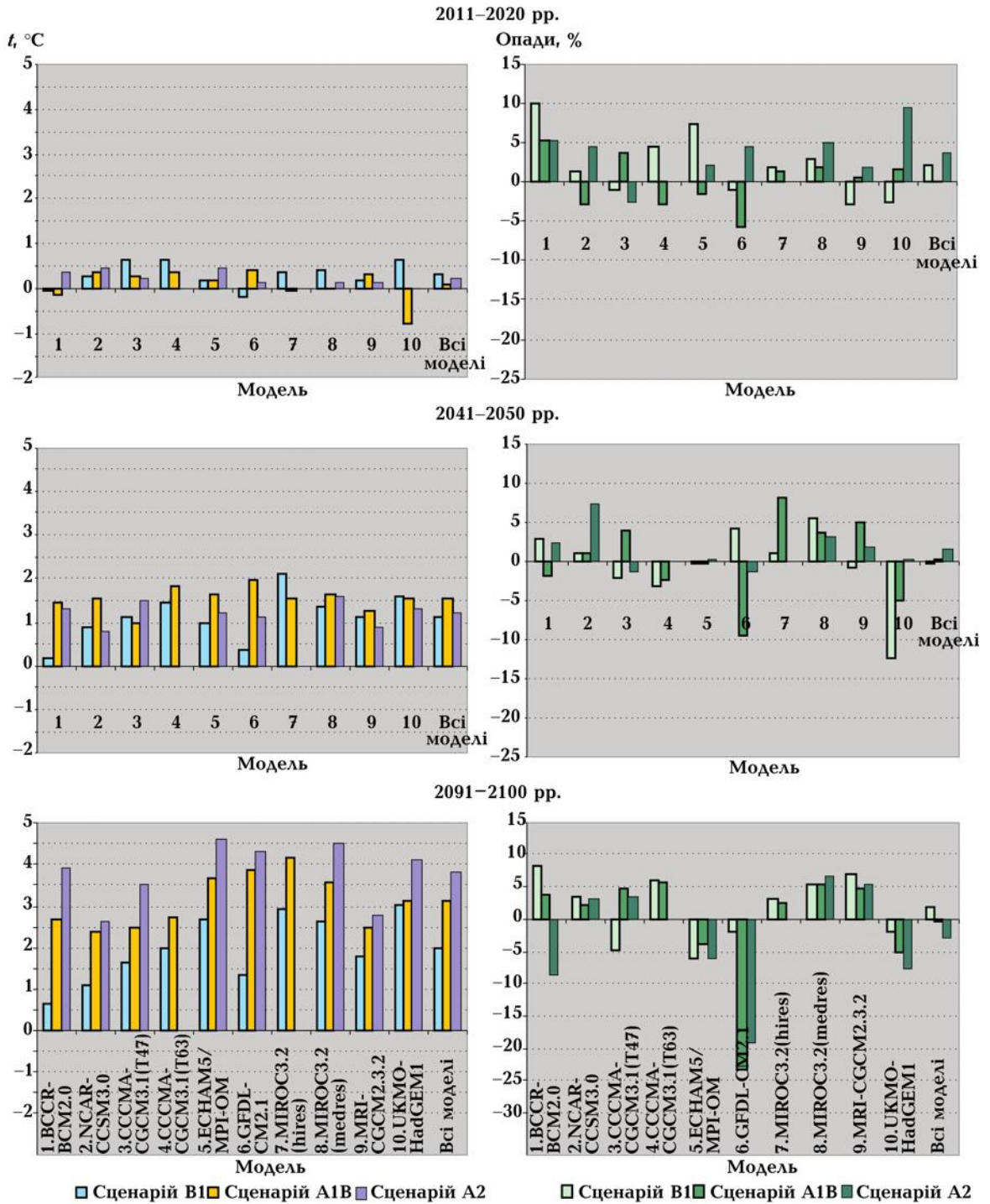
Рис. 4. Зміна середньорічних температур повітря (а) та кількості опадів (б) для різних сценаріїв у наступному, середньому та останньому десятиріччях XXI ст. порівняно з періодом 2001—2010 рр.
