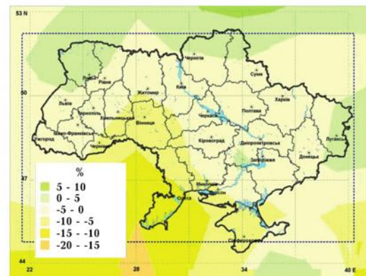
Рис. 5. Зміна в Україні річних температур повітря (а) і кількості опадів, % (б), середніх за десятиріччя XXI ст., порівняно з періодом 2001—2010 рр. Дані ансамблю 4 розрахунків моделі ECHAM5/MPI-OM за сценарієм А1В.
