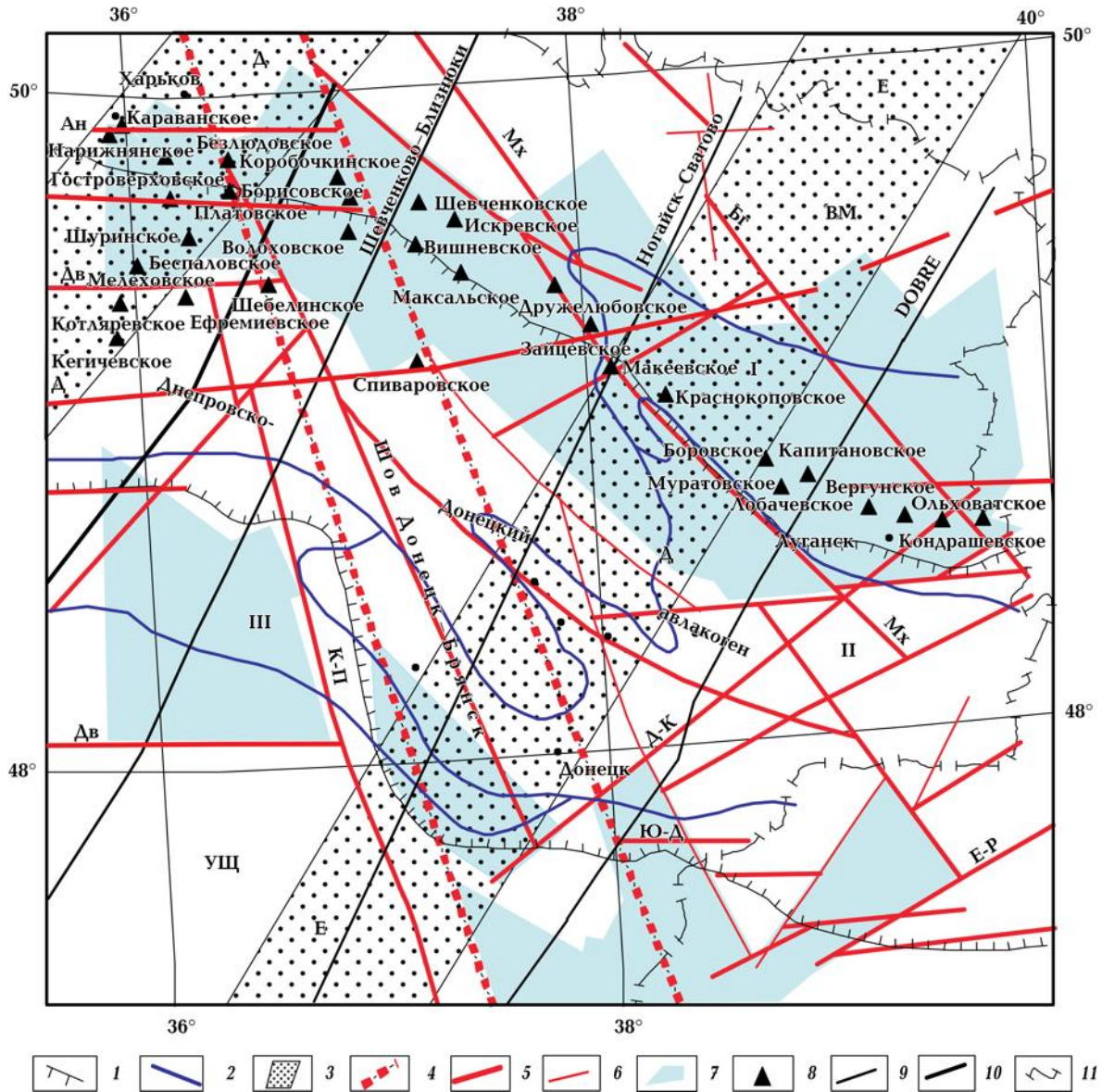
Рис. 1. Схема основных разломов консолидированной коры, литосферных линеаментов и газоносности юго-восточной части ДДд в сопоставлении с намагниченностью пород консолидированной коры: 1 — граница ДДд; 2 — границы районов Донбасса (I — северный, II — складчатый, III — западный); 3 — литосферные линеаменты Д и Е, по [Сологуб, 1986]; 4 — трансрегиональный тектонический шов Донецк—Брянск (Д-Бр); 5 — разломы I порядка; 6 — разломы более высоких порядков; 7 — проекции глубинных магнитных блоков на земную поверхность; 8 — месторождения газа; 9 — профили ГСЗ; 10 — профиль «Эталонный Шебелинский»; 11 — государственная граница Украины. Главные разломы: Ц-Д — Центрально-Донецкий; Ю-Д — Южно-Донецкий; К-П — Криворожско-Павловский; Дв — Девладовский; Мх — Михайловский; Д-К — Донецко-Кадиевский; Е-Р — Еланчикско-Ровенковский; Бг — Белгородский; Ан — Андрушевский.
