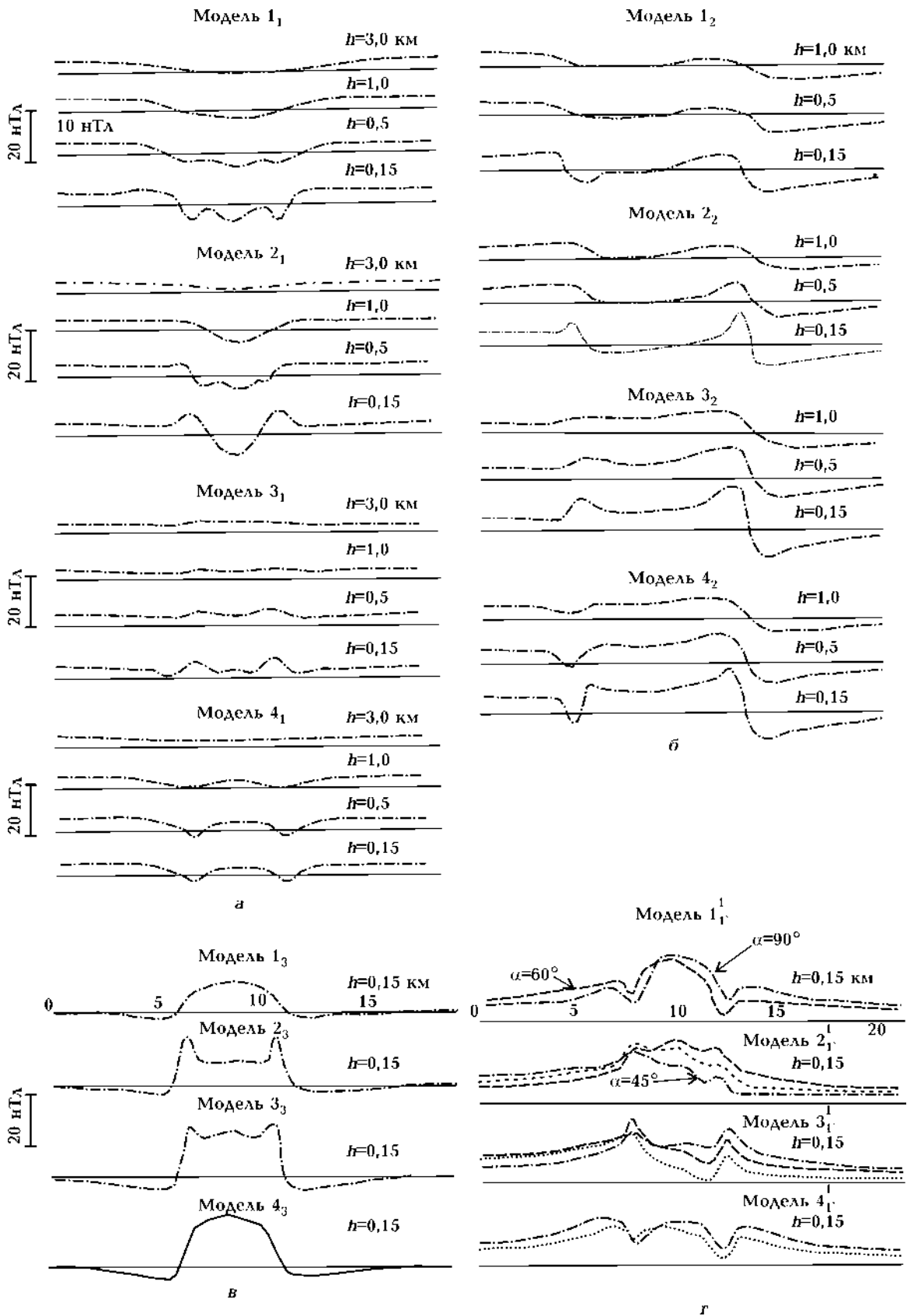
Рис. 4. Поле (\Delta T)_a , рассчитанное для разных моделей нефтегазонасыщенной структуры: а — 1_1 \div 4_1 ; б — 1_2 \div 4_2 ; в — 1_3 \div 4_3 ; г — 1_г \div 4_г .
