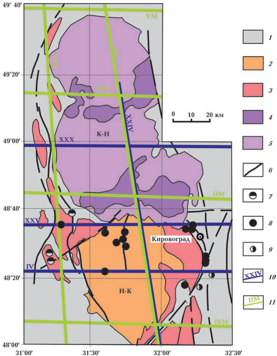
Рис. 5. Сейсмическая изученность Кировоградского рудного района: 1 — ингуло-ингулецкая серия; 2, 3 — Новоукраинско-Кировоградский массив (Н-К) (2 — диорит-монцитовая формация; 3 — гранит-мигматитовая формация); 4, 5 — Корсунь-Новомиргородский массив (К-Н) (4 — габбро-анортозитовая формация; 5 — рапакиви-гранитная формация); 6 — разломы; 7—9 — месторождения и рудопроявления (7 — лития, 8 — урана, 9 — золота); 10 — профили ГСЗ и их номера; 11 — профили МОВЗ и их номера.
