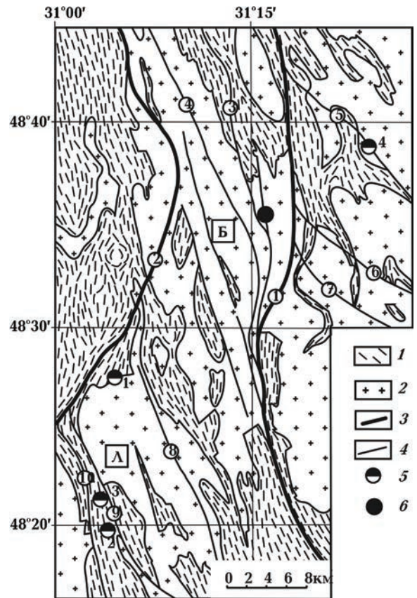
Рис. 1. Схематическая геологическая карта Звенигородской зоны разломов. Составлена по материалам КП "Кировгеология" с использованием государственной геологической карты масштаба 1 : 200 000 [Державна ..., 2001]: 1, 2 — интрузивно-ультраметаморфический цоколь (1 — метаморфические породы ингуло-ингулецкой серии, 2 — гранитоиды кировоградского комплекса); 3, 4 — наложенные структуры (3 — разломы I порядка, 4 — разломы II порядка); 5, 6 — месторождения (5 — лития (1 — Липняжское, 2 — Надия, 3 — Станковатское, 4 — Полоховское), 6 — Ватутинское урановое месторождение). Массивы гранитоидов (буквы в квадратах): Б — Березовский, Л — Липняжский. Разломы (цифры в кружках): 1 — Новопавловский, 2 — Марковский, 3 — Восточно-Курниковский, 4 — Западно-Курниковский, 5 — Копанский, 6 — Хмелевский, 7 — Калиновский, 8 — Добровеличковский, 9 — Маловильшанский, 10 — Станковатский.
