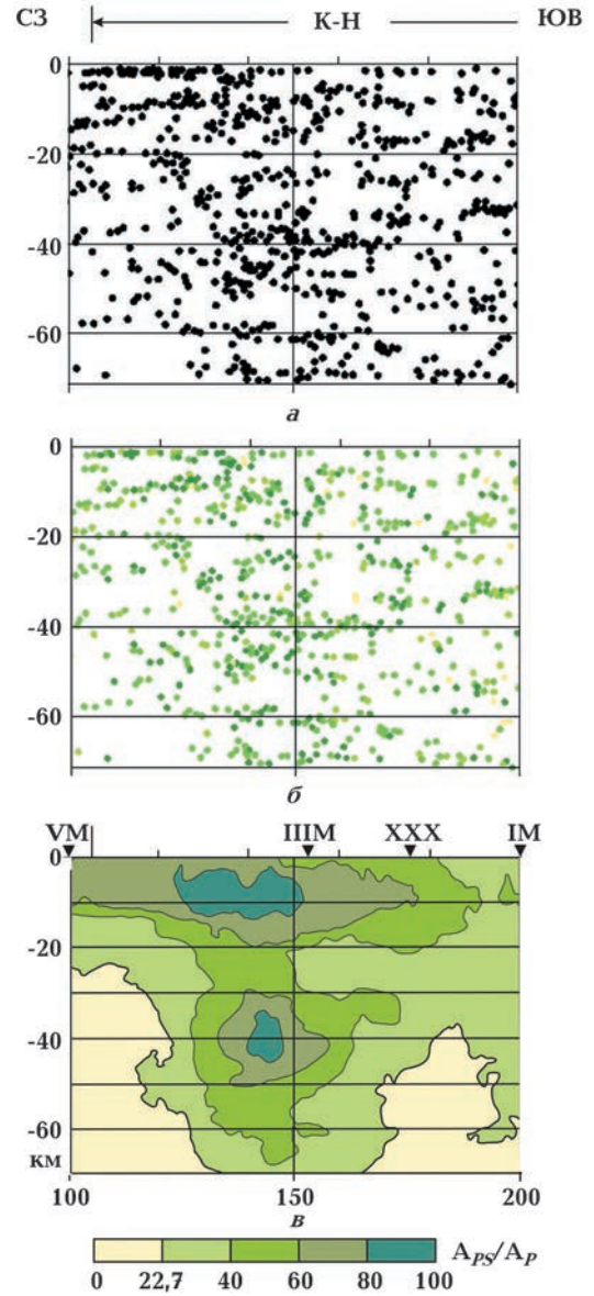
Рис. 6. Трансформация поля обменных волн. Фрагмент профиля ИМ: а — исходное поле обменов; б — распределение параметра A_{PS}/A_P в тех же точках; в — результат осреднения параметра A_{PS}/A_P в изометрическом окне ( R = 11,5 км).
