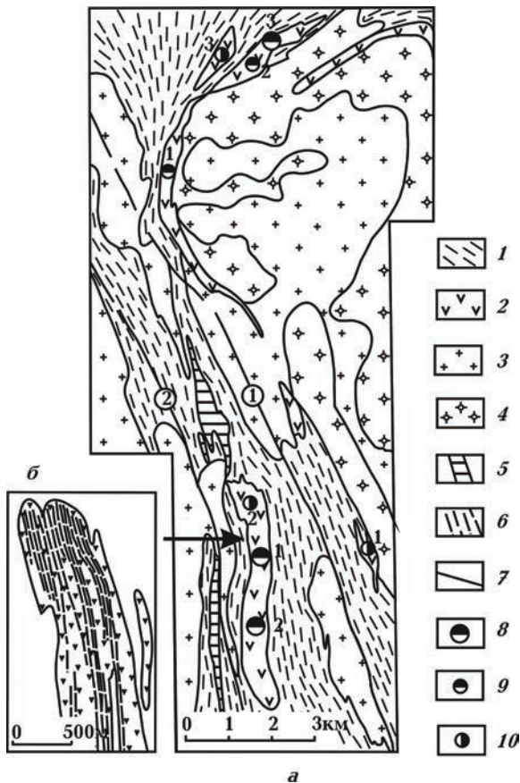
Рис. 2. Схематические геологические карты Станковатского рудного поля (а) и Станковатского пегматитового литиевого месторождения (б): 1, 2 — ингуло-ингулецкая серия (1 — гнейсы, 2 — амфиболиты); 3—5 — кировоградский интрузивный комплекс (3 — биотитовые граниты, 4 — биотитовые мигматиты, 5 — двуполовшатовые пегматиты); 6 — редкометалльные пегматиты; 7 — разломы (1 — Маловильшанский, 2 — Станковатский); 8 — литиевые месторождения (1 — Станковатское, 2 — Надя, 3 — Липняжское); 9 — редкометалльные рудопроявления (1 — Новоодесское, 2 — Скарновое); 10 — рудопроявления золота (1 — Контактное, 2 — Станковатское, 3 — Овражное).
