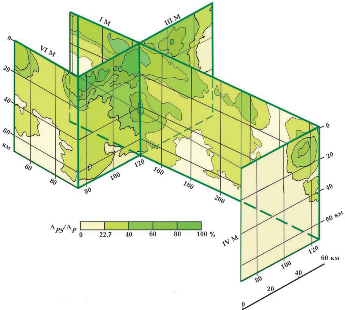
Рис. 7. Каркасная блок-диаграмма распределения параметра A_{PS}/A_P .
