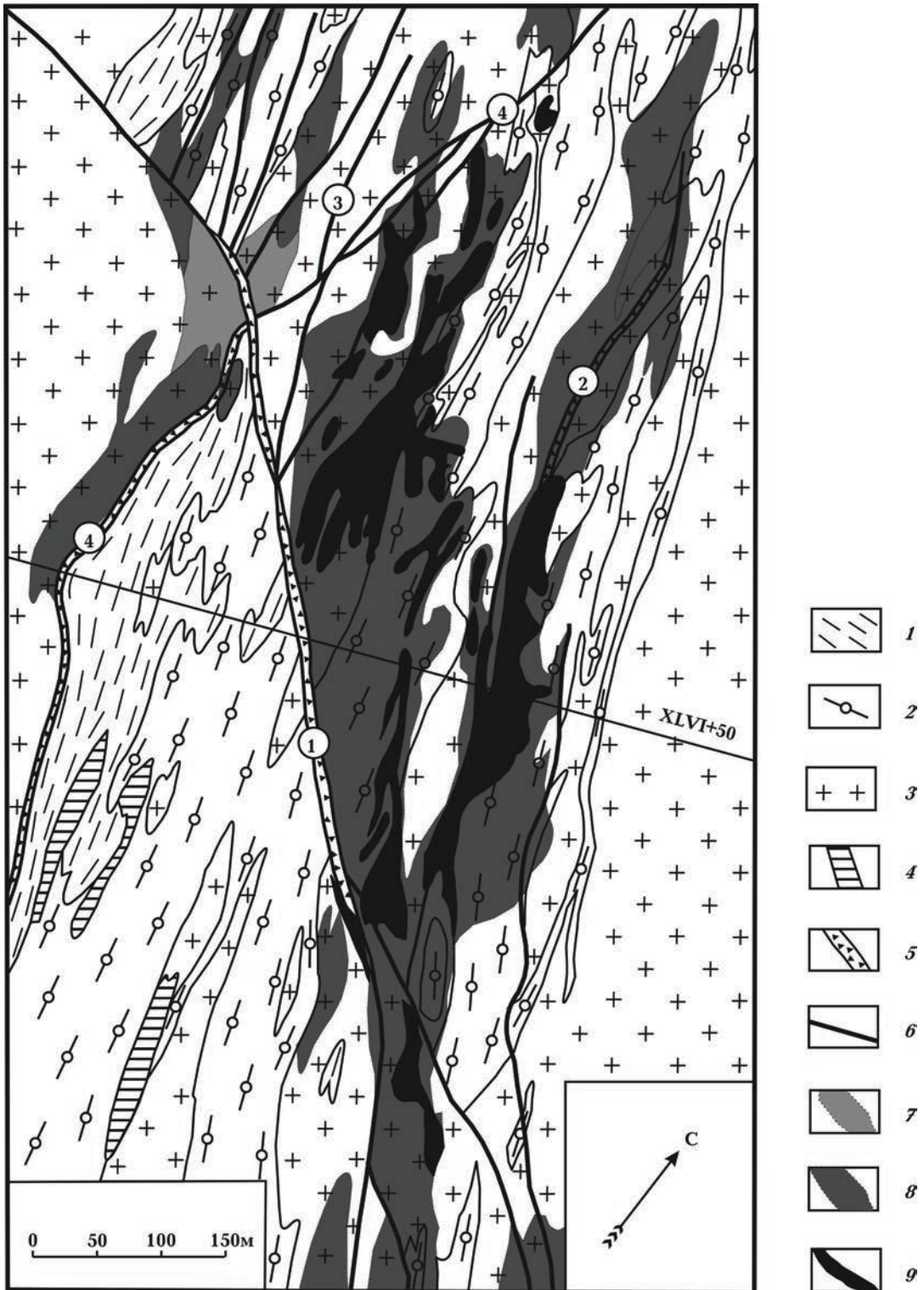
Рис. 3. Геологический план горизонта –115 м Ватутинского уранового месторождения, по [Генетические ..., 1995] с изменениями: 1 — гнейсы; 2 — мигматиты; 3, 4 — граниты (3 — среднезернистые, 4 — пегматоидные); 5, 6 — разрывные нарушения (5 — в масштабе, 6 — вне масштаба); 7, 8 — натровые метасоматиты (7 — десилицированные породы, 8 — альбититы), 9 — рудные тела. Названия разломов (цифры в кружках): 1 — Главный западный, 2 — Восточный, 3 — Меридиональный, 4 — Пологий.
