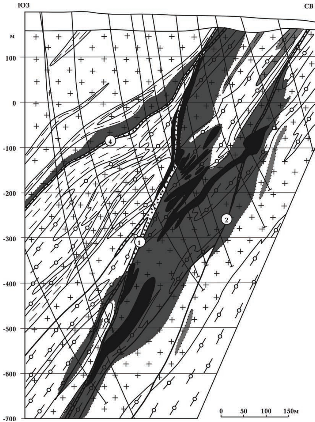
Рис. 4. Геологический разрез Ватуhtинского уранового месторождения по разведочной линии XLVI-50, по [Генетические ..., 1995] с изменениями. Условные обозначения см. на рис. 3.
