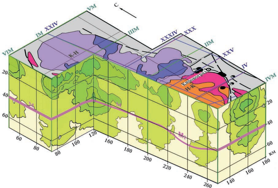
Рис. 8. 3D сейсмогеологическая модель Кировоградского рудного района: М — раздел Мохо, M_P — мантийный ров. Остальные условные обозначения см. на рис. 5 и 7.
