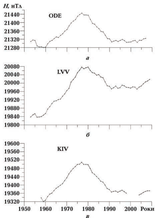
Рис. 1. Середньорічні значення H -компоненти за всіма днями на геомагнітних обсерваторіях "Одеса" (ODE), "Львів" (LVV) і "Київ" (KIV): a — 1953—2007 рр.; b — 1953—2009 рр.; v — 1958—2009 рр.
