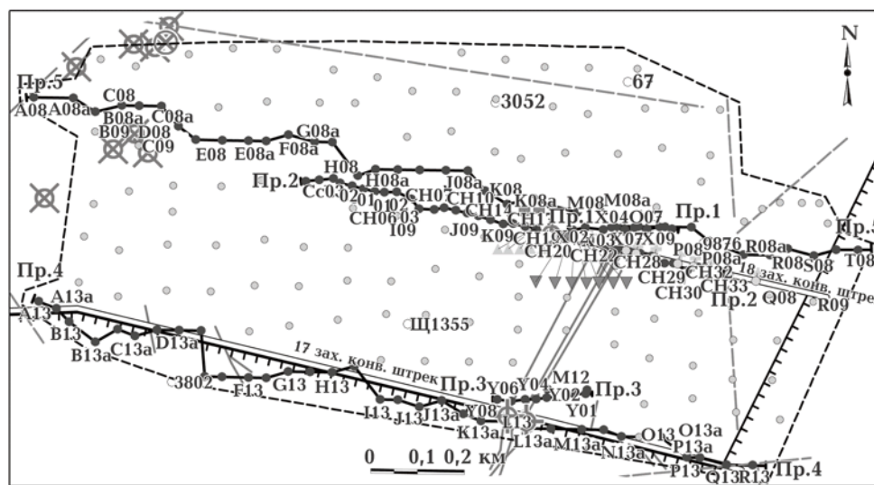
Рис. 2. Карта і план просторового розташування ділянок і пунктів спостереження СТАГД у межах гірничого відводу шахти ім. О. Ф. Засядька: 1 — ділянки СТАГД та їх номери (I — «Північна», II — деталізаційних досліджень); 2 — профілі спостережень та їх номери; 3 — пункти спостережень СТАГД (а — площинних, б — профільних); 4 — пункти атмогеохімічних досліджень у гірничій виробці (18 західний конвеєрний штрек) (а — відбір проб газу у повітрі штреку, б — відбір проб газу із стінок штреку, в — дегазаційні свердловини, із яких відбирали проби газу та їх номери, г — відбір проб вугілля для вакуумної дегазації, д — відбір проб шламу із дегазаційної свердловини); 5 — лінементи за даними МАКЗ; 6 — свердловини та їх номери; 7 — шахтний стовбур; 8 — тектонічне порушення за даними св. 3985; 9 — умовні позначення з плану гірничих робіт по пласту n_1 (а — очікуваний насув, б — насуви, в — осередки ліквідованих пожеж, г — місця вибуху газу); 10 — умовні позначення з плану гірничих робіт по пласту m_3 (а — розривні порушення та зони тріщинуватості за результатами проходки, б — межа відпрацьованої частини пласта, в — проходка станом на 05.2009 18-й і 17-й західні конвеєрні штреки, г — місця раптових викидів газу, вугілля, порід); 11 — межа шахтного поля шахти ім. О. Ф. Засядька.
