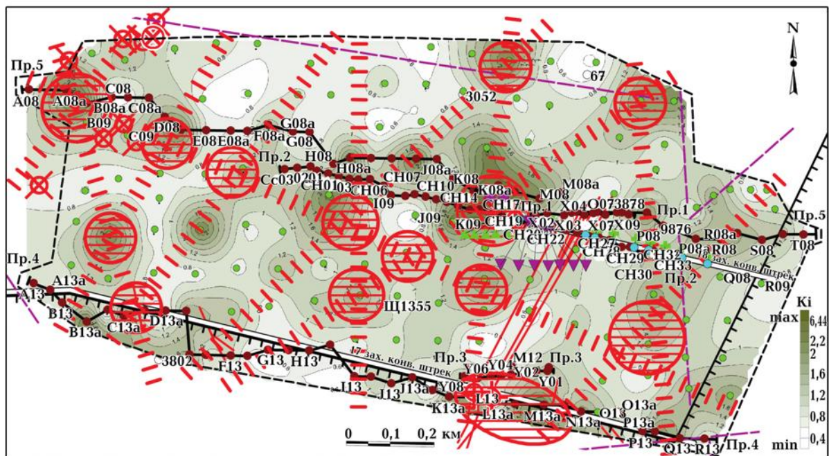
Рис. 5. Карта зон тріщинуватості та розуцільнення гірських порід, ділянок можливих проявів ГДЯ на ділянці деталізаційних досліджень (на основі карти розподілу показників значень та інтегрального коефіцієнта K_i ).
