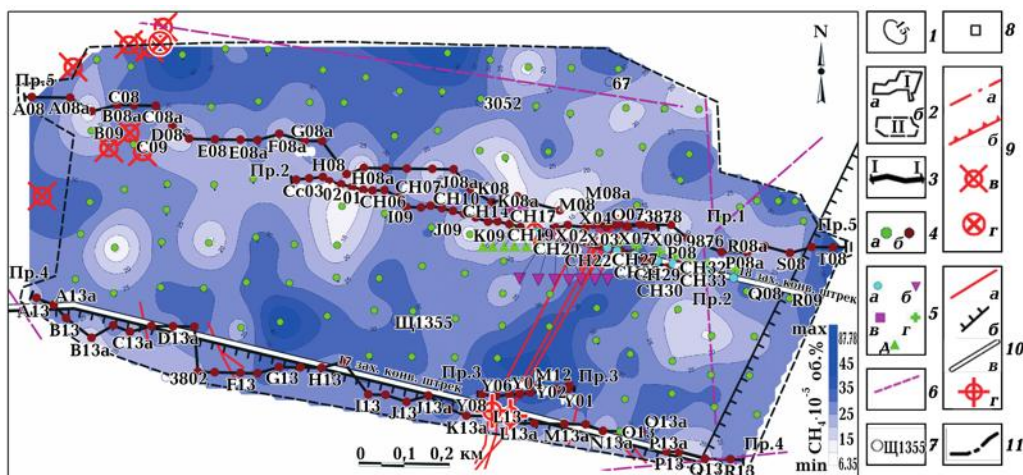
Рис. 3. Карта розподілу показників вмісту метану ( CH_4 \cdot 10^{-5} \% ) у підґрунтовому шарі повітря: 1 — ізолінії показників вмісту метану; 2 — межа ділянки деталізаційних досліджень; 3 — профілі спостережень та їх номери; 4 — пункти спостережень СТАГД (а — площинних, б — профільних); 5 — пункти атмогеохімічних досліджень у гірничій виробці (18 західний конвеєрний штрек) (а — відбір проб газу у повітрі штреку, б — відбір проб газу із стінок штреку, в — дегазаційні свердловини, із яких відбирали проби газу та їх номери, г — відбір проб вугілля для вакуумної дегазації, д — відбір проб шламу із дегазаційної свердловини); 6 — лінеamenti за даними МАКЗ; 7 — свердловини та їх номери; 8 — шахтні стводи; 9 — умовні позначення з плану гірничих робіт по пласту n_1 (а — очікуваний насув, б — насиви, в — осередки ліквідованих пожеж, г — місця вибуху газу); 10 — умовні позначення з плану гірничих робіт по пласту m_3 (а — розривні порушення та зони тріщинуватості за результатами проходки, б — відпрацьованої частини пласта, в — проходка станом на 05.2009 18-й і 17-й західні конвеєрні штреки, г — місця раптових викидів газу, вугілля, порід); 11 — межа шахтного поля шахти ім. О. Ф. Засядька.
