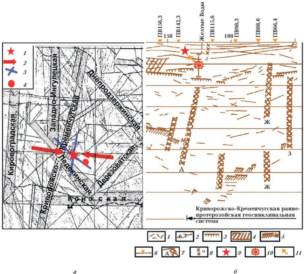
Рис. 12. Сейсмотектоническая позиция очага Криворожского землетрясения: а — фрагмент тектонической карты Украины по работе [Єнтін, 2005] (1 — эпицентр Криворожского землетрясения 25.12.2007 г., 2 — направления осей сжатия, 3 — пространственное положение нодальных плоскостей, 4 — эпицентр землетрясения 2001 г.); б — фрагмент сейсмогеологического разреза по профилю VIII Таганрог — Днепропетровск — Могилев-Подольский, Голованевск — Винница по работе [Строение ..., 1978] (1 — отражающие площадки, 2 — линии изоскоростей в кристаллической толще, км/с, 3 — протяженные отражающие горизонты в кристаллической толще, 4 — слой с пониженной скоростью в кристаллической толще, 5 — отражающие границы раздела М, 6 — пункты взрыва, 7 — глубинные и другие крупные разломы по данным ГСЗ (А — Криворожско-Кременчугский, Ж — Верховцевский, З — Криничанский), 8 — разломы по геологическим данным (∂ — Криворожско-Кременчугский), 9, 10 — макросейсмический и инструментальный гипоцентры соответственно, 11 — направление вспарывания разрыва.
