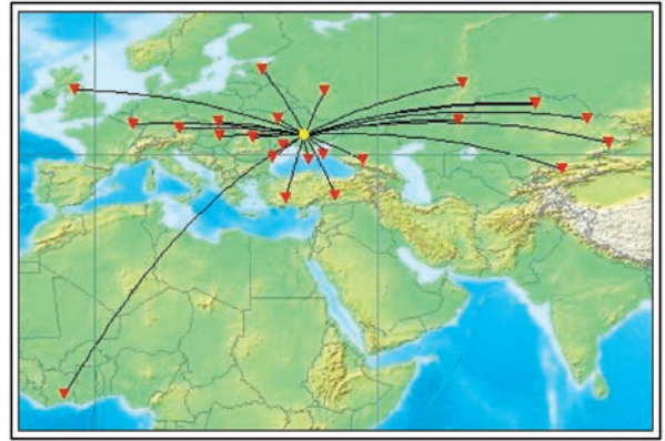
Рис. 3. Географическое расположение сетей сейсмических станций, данные которых использованы в настоящей работе. Сплошными линиями обозначены кратчайшие расстояния до эпицентра по поверхности земной сферы.
