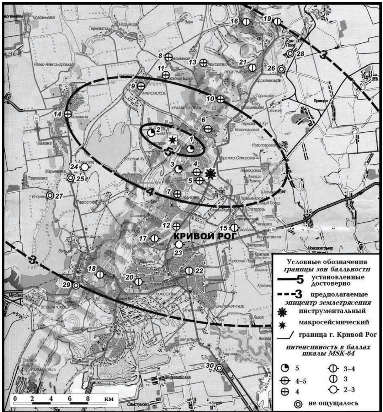
Рис. 7. Схема распределения макросейсмического эффекта Криворожского землетрясения 25 декабря 2007 г. Составили: Скляр А.М., Князева В.С. Значок интенсивности соответствует центру территории, для которой определялась интенсивность сотрясений.
