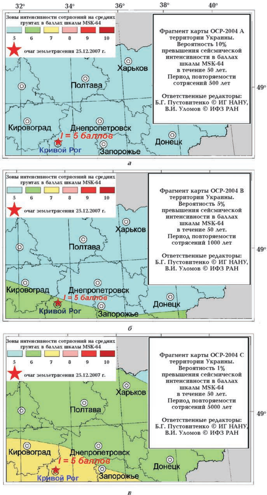
Рис. 1. Долговременная сейсмическая опасность района землетрясения 25.12.2007 г. для периодов повторяемости: a — 500 лет, б — 1000 лет, в — 5000 лет [Пустовитенко и др., 2006]. Звездочкой отмечен эпицентр произошедшего землетрясения с указанием интенсивности в эпицентре.
