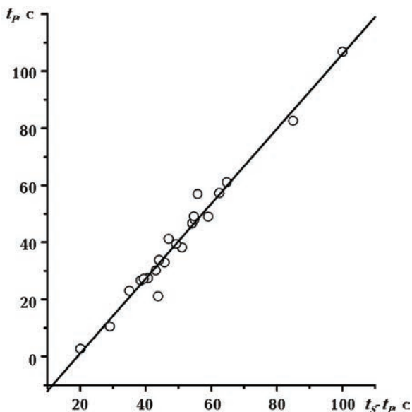
Рис. 6. График Вадати для Криворожского землетрясения 25 декабря 2007 г.
