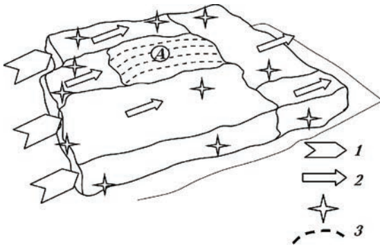
Рис. 11. Объемная модель системы подготовки землетрясения при движении блоков под действием тектонических сил: 1 — общее направление движения всей системы блоков; 2 — направление движения отдельного блока; 3 — землетрясения малого энергетического класса; 4 — деформация растяжения, возникающая при остановке блока А.
