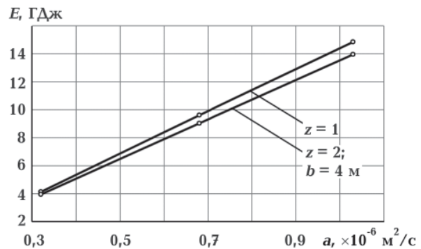
Рис. 4. Залежність ефективної теплової енергії за час функціонування теплообмінника від теплопровідності ґрунту.
