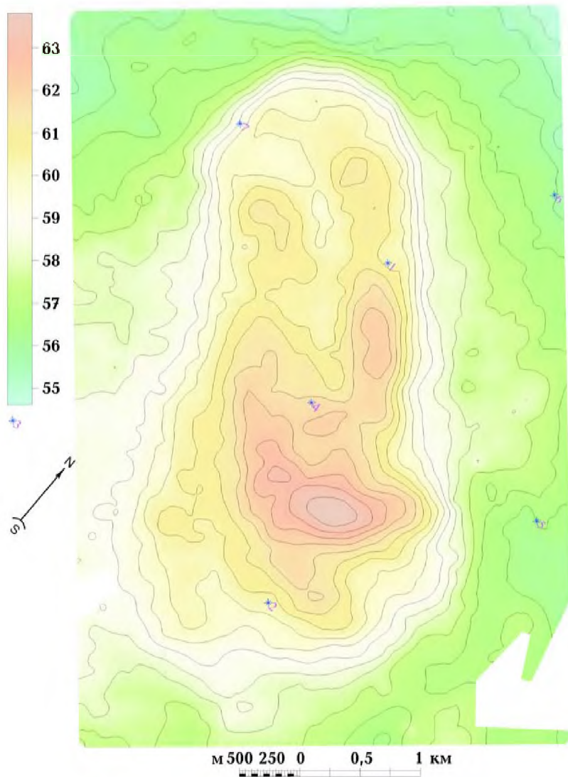
Рис. 3. Карта изоаномал силы тяжести Тарасовского участка по материалам гравиметрической съемки 1 : 10 000. Редукция Буге, \sigma = 2,3 \text{ г/см}^3 . Сечение изоаномал 0,5 мГал.
