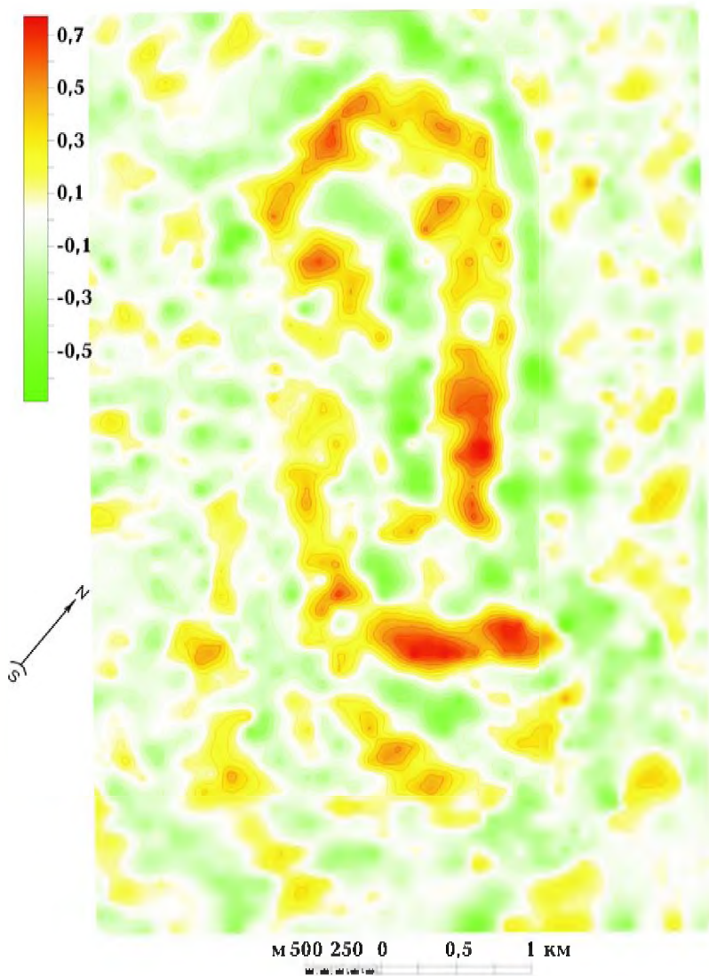
Рис. 4. Карта локальных аномалий силы тяжести Тарасовского участка по материалам гравиметрической съемки 1 : 10 000. Сечение изолиний \delta\Delta g 0,1 мГал.
