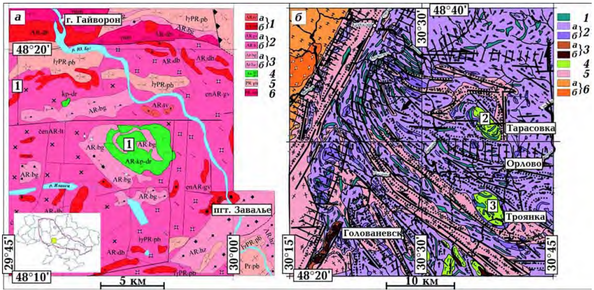
Рис. 1. Положение Бандуровского (1), Тарасовского (2) и Троянского (3) базитовых массивов в геологической структуре ПГРР: a — фрагмент геологической карты м-ба 1 : 200 000 кристаллического фундамента листа М-35-XXXVI-Гайворон, по [Зюльце та ін., 2002] (1 — кристаллические сланцы и плагиогнейсы амфибол-пироксеновые, кварциты пироксен-магнетитовые (днепровско-бугская серия) ( a ); кристаллосланцы и плагиогнейсы пироксеновые, часто амфиболлизированные и кристаллосланцы амфиболитовые (днепровско-бугская серия нерасчлененная) ( b ); 2 — эндербиты гнейсоподобные (en 1 ) (гайворонский ультраметаморфический комплекс) ( a ); чарнокиты, чарноэндербиты, эндербиты с телами лейкократовых гранитов (cen) (литинский ультраметаморфический комплекс) ( b ); 3 — кристаллосланцы и плагиогнейсы пироксеновые, часто с амфиболами, иногда с гранатом, плагиогнейсы биотитовые, графит-биотитовые, иногда с силлиманитом и кордиеритом, кварциты, кальцифиры, плагиогнейсы амфибол-биотитовые и амфиболиты (бугская серия нерасчлененная) ( a ); кальцифиры, плагиогнейсы биотит-графитовые (часто с гранатом и (или) силлиманитом, (бугская серия, хщевато-завальевская свита) ( b ); 4 — габброиды амфиболитовые, габбро-амфиболиты, апогабброидные кристаллосланцы (капитановско-деренюхинский интрузивный комплекс); 5 — граниты и гранитоиды лейкократовые с ортопироксеном, часто с гранатом, иногда с кордиеритом (lr) (побужский ультраметаморфический комплекс); 6 — граниты биотитовые средне-крупнозернистые до порфировидных ( r ), граниты и мигматиты биотитовые, равномерно зернистые (gm) (уманский ультраметаморфогенный комплекс)); b — фрагмент структурно-петрофизической основы геологической карты м-ба 1 : 100 000 кристаллического фундамента центральной части ГШЗ (лист М-36-XXXI-Первомайск), по [Гинтов и др., 2016] (1 — кристаллосланцы дупироксеновые, ортопироксеновые, биотит-ортопироксеновые, гранат-ортопироксеновые, магнетит-дупироксеновые; 2 — эндербиты, чарнокиты с мелкими включениями кристаллосланцев дупироксен-плагиоклазовых и розовых гранитов — чарнокиты, часто гранатсодержащие ( a ); эндербиты, чарнокиты с крупными включениями кристаллосланцев дупироксен-плагиоклазовых и розовых гранитов — эндербито-гнейсы ( b ); 3 — плагиогнейсы, гнейсы гранат-биотитовые, кварциты полевошпатовые (часто с силлиманитом, кордиеритом и гранатом), кристаллосланцы и плагиогнейсы пироксеновые ( a ); гнейсы биотит-графитовые, кальцифиры доломит-кальцитовые, кальцитовые, кварциты железистые, в основном магнетит-дупироксеновые, кальцифиры магнетитовые рудные ( b ); 4 — метагабброиды — амфиболиты, габбро, габбро-амфиболиты; серпентиниты, серпентинизированные ультрабазиты; 5 — розовые и серовато-розовые полосчатые гранат-биотитовые гнейсо-граниты, редко массивные побужского (чуднобердичевского) комплекса, гнейсо-граниты полосчатые розовые и серовато-розовые, как правило, динамометаморфически измененные синицовского комплекса; 6 — серые и розовато-серые граниты биотитовые, неравномернозернистые до порфировидных уманского комплекса ( a ); плагиограниты амфибол-биотитовые, иногда с гранатом, ортопироксеном гайсинского комплекса ( b ). Условные обозначения сокращения: охарактеризованы только вещественные комплексы, пронумерованные под обеими картами по максимально возможной сопоставимости друг с другом.
