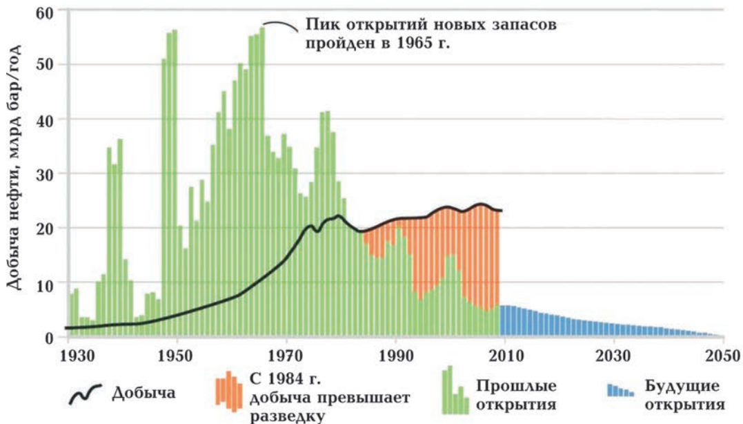
Рис. 1. Графики производства (добычи) и воспроизводства (открытий): а — мировое производство сырой нефти и конденсата, включая ведущие страны-производители нефти до 2050 г. (www.peakoil.net), б — мировые открытия (www.aspo-ireland.org).
