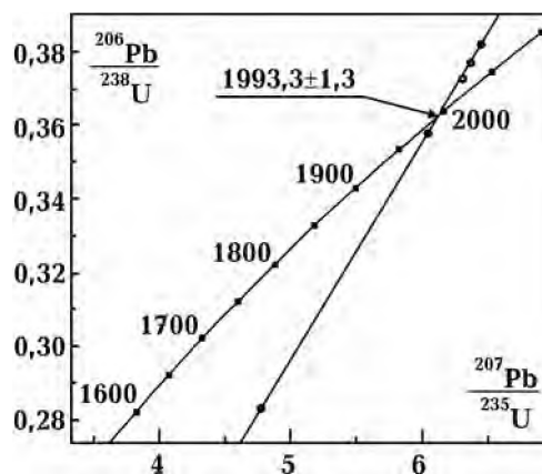
Рис. 11. U-Pb диаграмма с конкордией для монацита из кварц-гранат-двуполевошпатовой породы (метасоматита), проба SB-5-1, левый берег р. Южный Буг, южная окраина с. Хащеватое.
