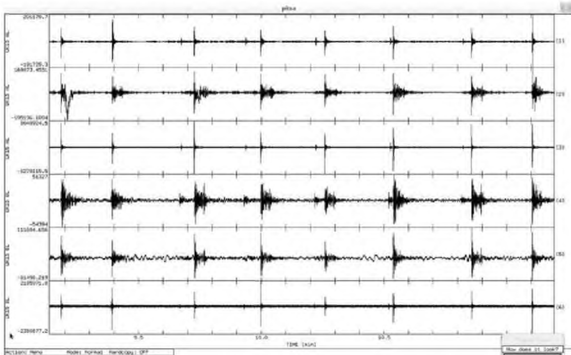
Рис. 1. Шість поканальних потоків сейсмоакустичної інформації, записані датчиками, кожен з яких реєструє сейсмічні та акустичні коливання одночасно, отримані на полігоні «Дівичики» під час роботи міномета 82-го калібру.
