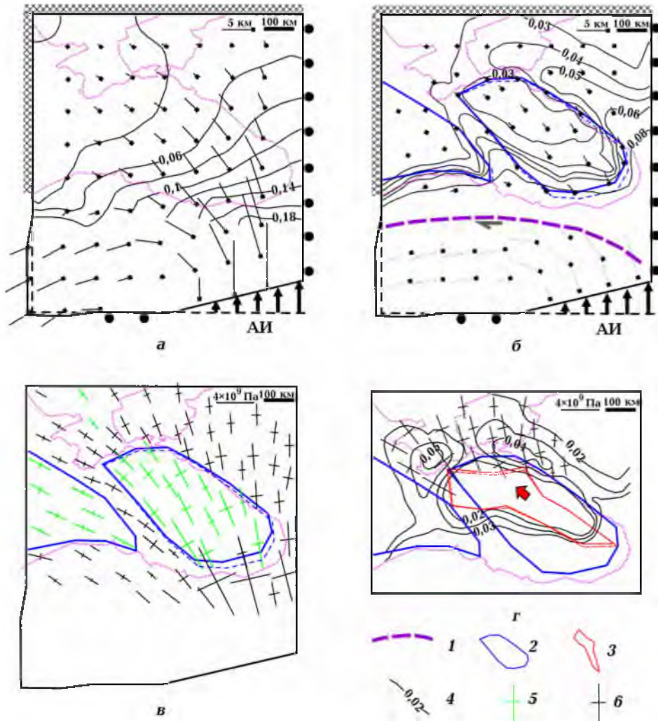
Рис. 5. Рассчитанные поля смещений, эквивалентных деформаций и напряжений в Восточно-Черноморском регионе при разных заданных условиях: a и б — поля смещений и деформаций в отсутствие упрочненных участков ( a ) и при введенных упрочненных участках-микроплитах, принадлежащих Западной и Восточной Черноморским впадинам ( б ). На рис. a показаны граничные условия, АИ — смещения Аравийского индентора; v и г — поля напряжений в присутствии упрочненных микроплит (стандартная схема, объясняющая появление Северо-Западного Кавказа) ( v ) и на северной границе ВЧМП вследствие движения локализованного индентора, оконтуривающего Алуштинско-Батумскую магнитную аномалию ( г ) (1 — условный тренд Северо-Анатолийского разлома; 2 — контур упрочненной плиты ВЧМП, штриховая линия — исходное положение; 3 — контур локализованного индентора внутри ВЧМП, штриховая линия — исходное положение; 4 — изолинии эквивалентной деформации; 5 и 6 — ориентировки главных нормальных напряжений в упругом (5) и пластическом (6) спектре деформаций). См. пояснения в тексте.
