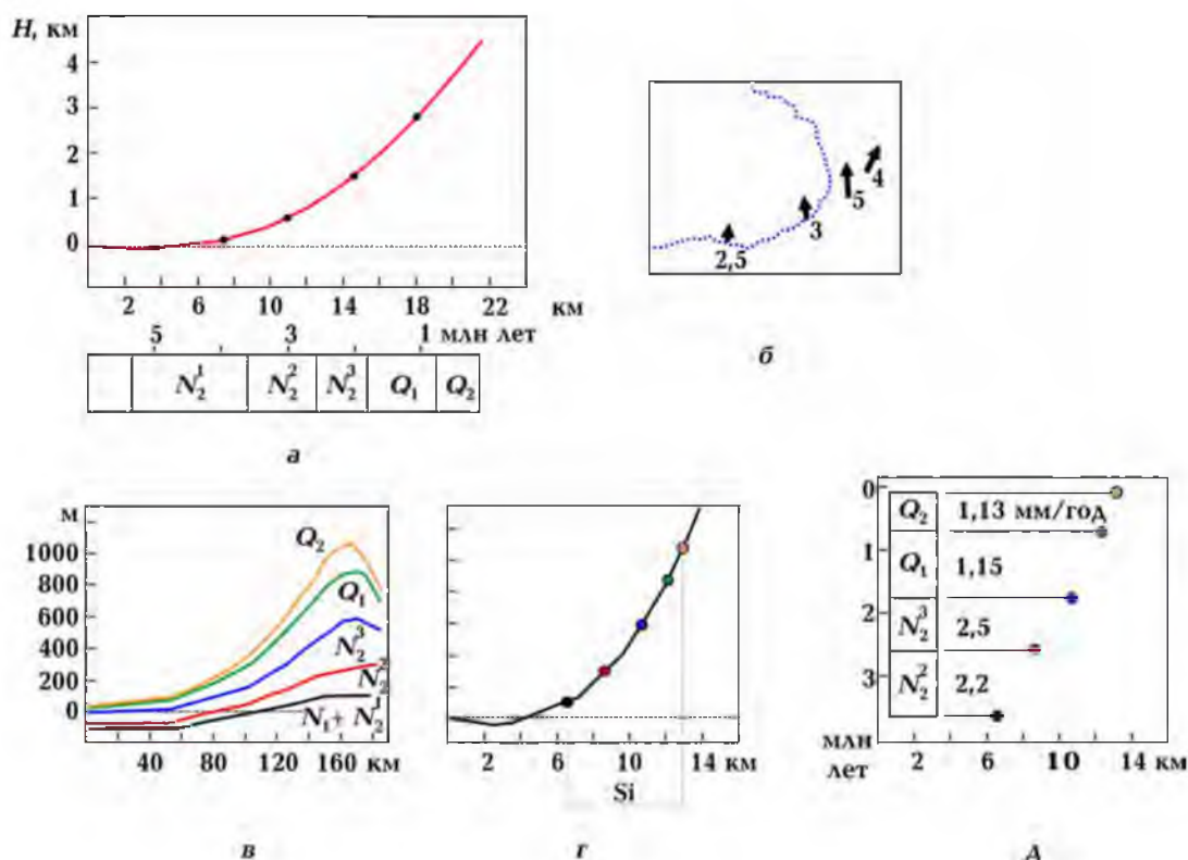
Рис. 11. Параметры вертикальных и горизонтальных движений при орогенезе на Центральном Кавказе и в Крыму: а — кривая вертикальных движений пика орогена в модели Центрального Кавказа; точками отмечены равные по времени интервалы, для которых определялась скорость вертикальных движений; б — векторы современных горизонтальных смещений поверхности вблизи юго-восточного побережья Черноморской впадины по GPS-данным [Reilinger et al., 2006] (цифры указывают величины скорости, мм/год); в — профили неотектонических движений вкост Центральной части Крыма для разных стратиграфических интервалов (с раннего плейстоцена по средний плейстоцен), составленные по данным [Бабак, 1961]; г — сопоставление интервальных значений подъема Горного Крыма с кривой вертикальных движений пика орогена в модели (аналогичной для Центрального Кавказа (рис. 11, а)); д — получаемая величина смещений индентора под Горным Крымом; д — интерпретация величин смещений индентора во временном масштабе; для соответствующих стратиграфических интервалов вынесены получаемые скорости.
