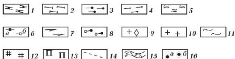
Рис. 9. Фрагмент геологической карты района Завальевского графитового месторождения (с сокращениями): Бугская серия. Хащевато-завальевская свита: 1 — кальцифиры, мраморы, карбонатные сланцы, 2 — гнейсы графитовые, гранат-биотит-графитовые, 3 — гнейсы биотитовые, гранат-биотитовые, 4 — гнейсы амфиболовые, 5 — скарноиды, 6 — кварциты (а — железистые, б — безрудные), 7 — амфиболиты; кошаро-александровская свита: 8 — гнейсы биотитовые, гранат-биотитовые, гранат-силлиманит-биотитовые, иногда с графитом; побужский комплекс: 9 — граниты аплит-пегматоидные, 10 — граниты биотитовые, 11 — мигматиты, 12 — чарнокиты, 13 — пироксениты; 14 — разломы, 15 — зоны дробления, 16 — буровые скважины (а — картировочные, б — глубокие наклонные). Звездочкой отмечено обнажение «Белая Скала» (см. рис. 10).
