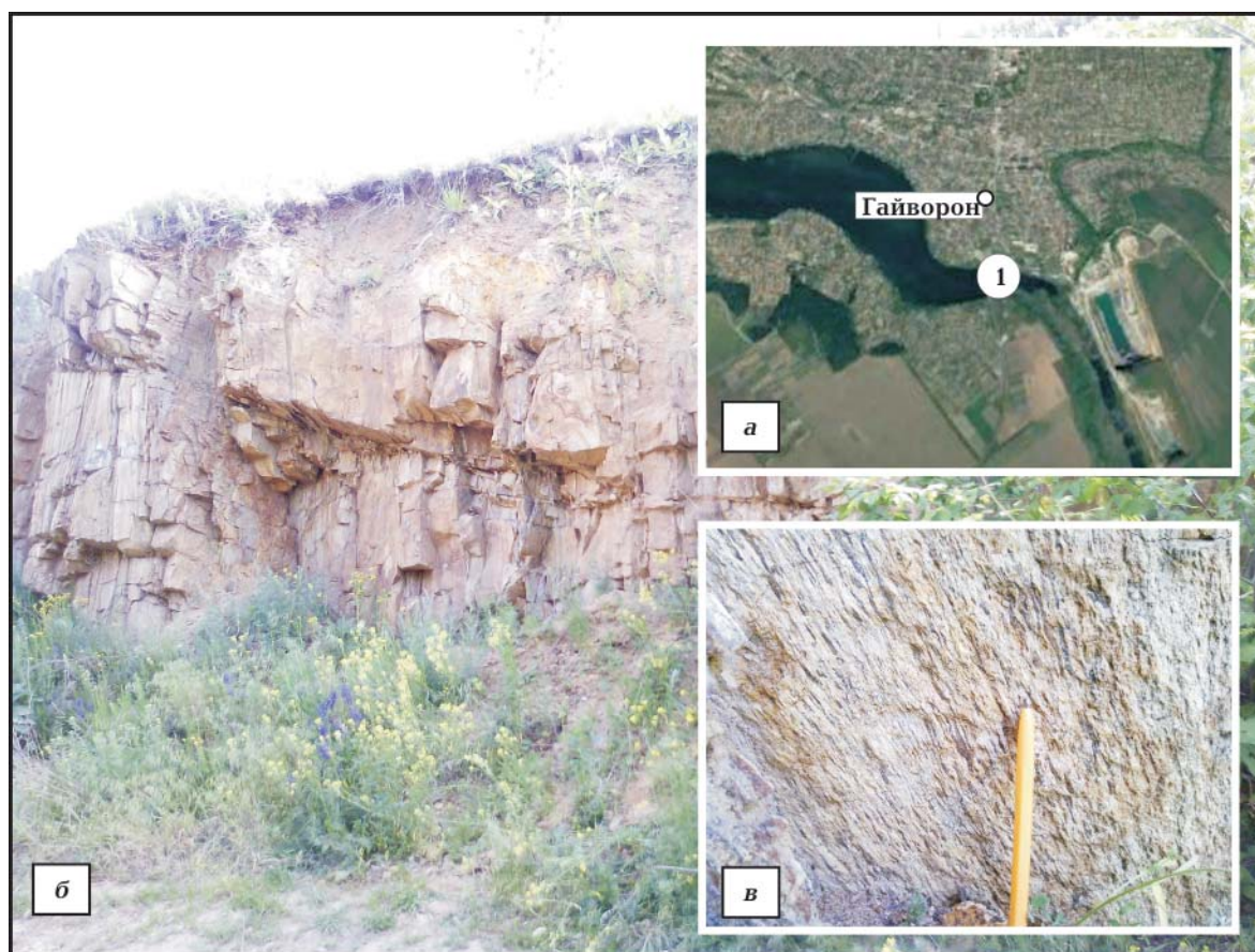
Рис. 4. Солгутовская зона скальвания. Обнажение эндербито-гнейсов на правом берегу р. Южный Буг: а — положение обнажения; б — общий вид обнажения; в — сланцеватость в эндербито-гнейсах. Фото А. В. Муровской.
