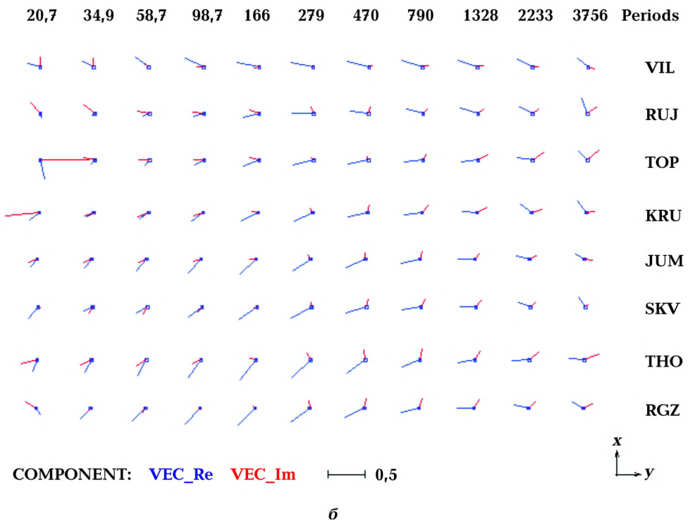
Рис. 2. Спостережені реальні та уявні компоненти типера за даними МВП для періодів геомагнітних варіацій від 20—30 до 3400—3700 с. Профілі: а — Радомишль—Фастів, б — Ружин—Сквира; RGZ — базовий МТ/МВ пункт спостереження Рогізна.
