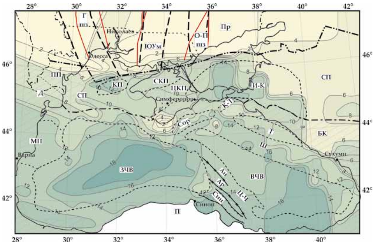
Рис. 7. Схема глубины залегания границы, которая одновременно является подошвой дислоцированных отложений и кровлей «гранитного» слоя. Штриховкой показаны области, в которых домеловые породы выходят на поверхность. Условные обозначения см. на рис. 1.
