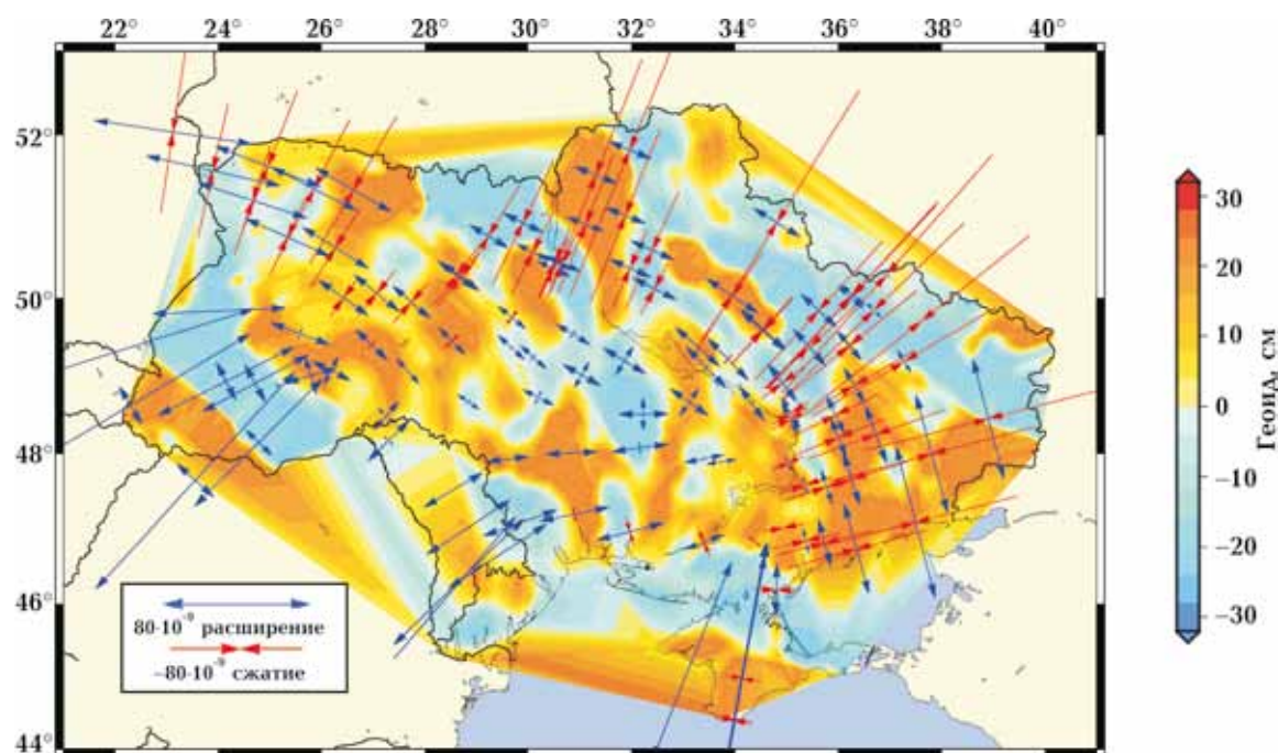
Рис. 5. Сравнительный анализ проявлений деформаций (эллипсы искривлений, синие стрелки — расширение, красные — сжатие) на примере «локального» квазигеоида УКГ2012лок.
