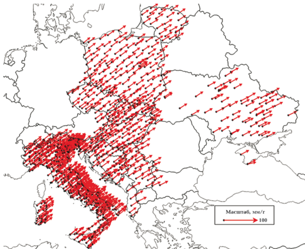
Рис. 2. Горизонтальная компонента векторов смещений ГНСС-станций для территории Центральной Европы, рассчитанная в рамках кампании SEGRN, система координат — IGB08.
