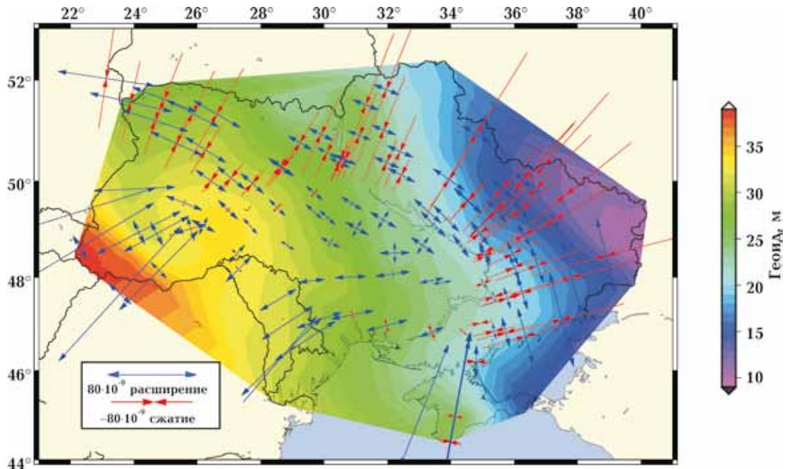
Рис. 3. Сравнительный анализ проявлений деформаций (эллипсы искривлений, синие стрелки — расширение, красные — сжатие) на примере «регионального» квазигеоида УКГ2012рег.
