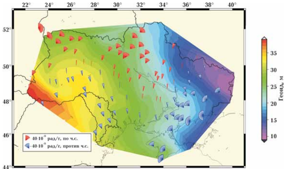
Рис. 4. Сравнительный анализ проявлений деформаций (вращения, красные радиусы по часовой стрелке, синие — против) на примере «регионального» квазигеоида УКГ2012рег.
