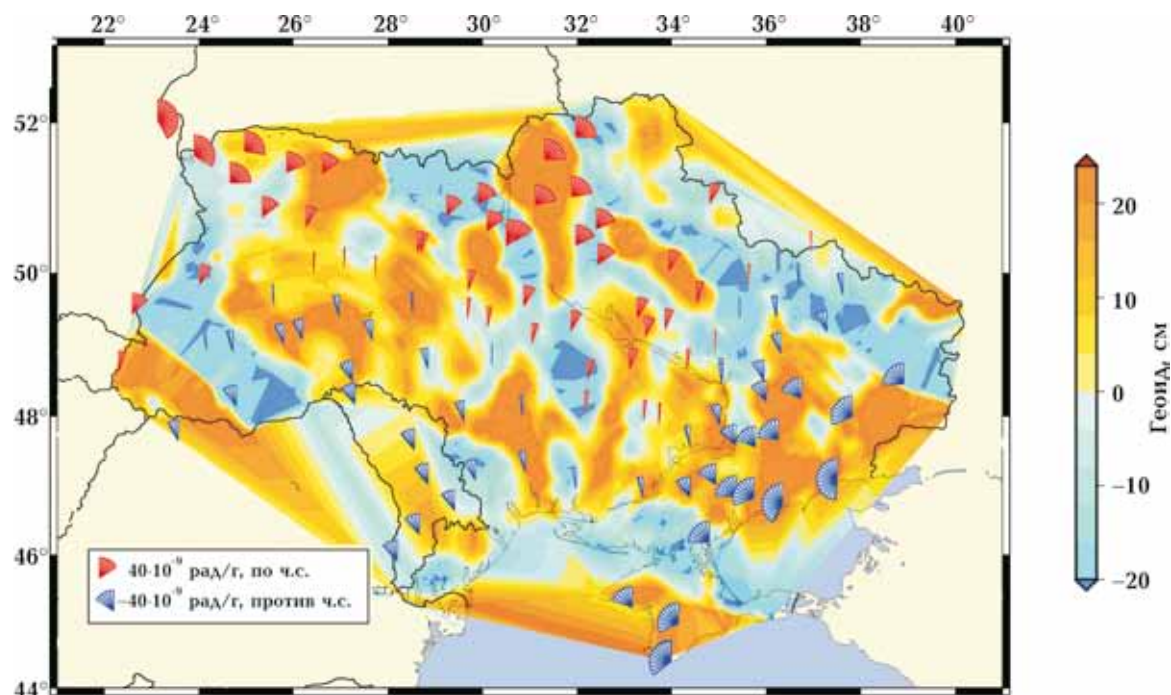
Рис. 6. Сравнительный анализ проявлений деформаций (вращения, красные радиусы — по часовой стрелке, синие — против) на примере «локального» квазигеоида УКГ2012лок.
