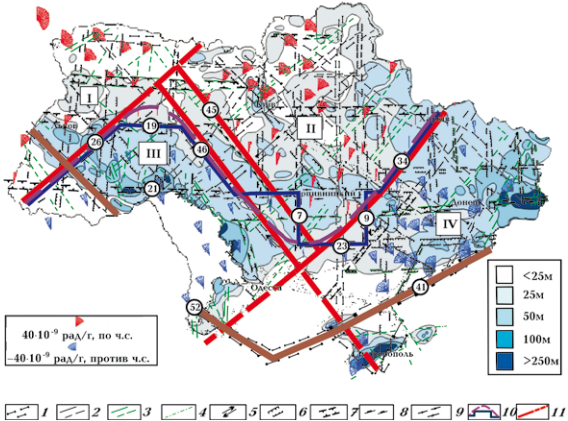
Рис. 8. Сопоставление аномалий деформаций поверхности Земли с новейшими движениями земной коры на примере вращения ее поверхности: 10 — варианты границ между областями лево- правостороннего вращения земной поверхности; 11 — предполагаемые границы между геоблоками земной коры. Цифры в кружках — номера линейментных зон (сохранена авторская нумерация [Верховцев, 2008]): 26 — Хустско-Корецкая, 19 — Яворовско-Волчанская, 46 — Камень-Каширско-Ялтинская, 45 — Ракитно-Новоархангельская, 21 — Мукачевско-Днепропетровская, 7 — Щорсовско-Николаевская, 23 — Баштанско-Тельмановская, 9 — Дружбинско-Орджоникидзевская, 34 — Магдалиновско-Мерефская, 41 — Сивашско-Каркинитская, 52 — Старосамборско-Змеиная. Другие условные обозначения см. на рис. 7.
