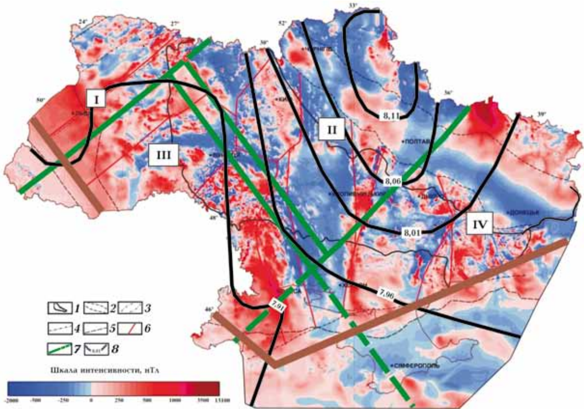
Рис. 9. Схема сопоставления современных геоблоков земной коры с геомагнитным полем \Delta T (по [Орлюк и др., 2015; Orlyuk et al., 2018]) и скоростями продольных сейсмических волн на глубине 50 км (по [Гейко и др., 1998]): 1—5 — границы Украинского щита (1); Днепровско-Донецкого авлакогена (2); Вольно-Оршанского рифта (3); трансрегиональные линеаменты края Восточно-Европейского кратона (по [Верховцев, 2008]) (4); (по [Bogdanova et al., 2016]) (5); 6 — зоны межмегаблоковых разломов; 7 — границы сочленения современных геоблоков земной коры; 8 — скорости продольных сейсмических волн на глубине 50 км (по [Гейко и др., 1998]).
