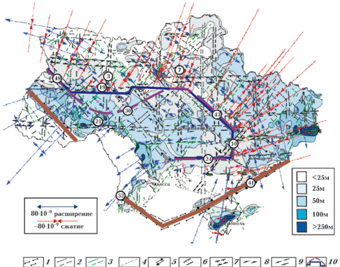
Рис. 7. Схема сопоставления аномалий деформаций поверхности Земли (эллипсов искривления) с новейшими движениями земной коры (составлена с использованием [Верховцев, 2008], для территории Закарпатья данные отсутствуют). Каркасные элементы линейментных зон: 1 — трансрегиональных, 2 — региональных 1-го порядка, 3 — то же 2-го порядка, 4 — одиночные линейменты; морфотипы линейментов: 5 — сдвиги, 6 — сбросы, 7 — взбросы, 8 — надвиги, 9 — раздвиги, 10 — варианты границ между областями преобладающего растяжения и сжатия земной поверхности.
