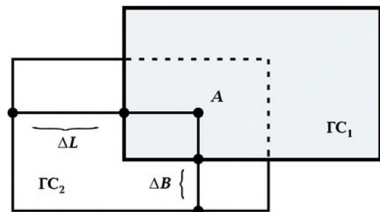
Рис. 5. Преобразование координат.
