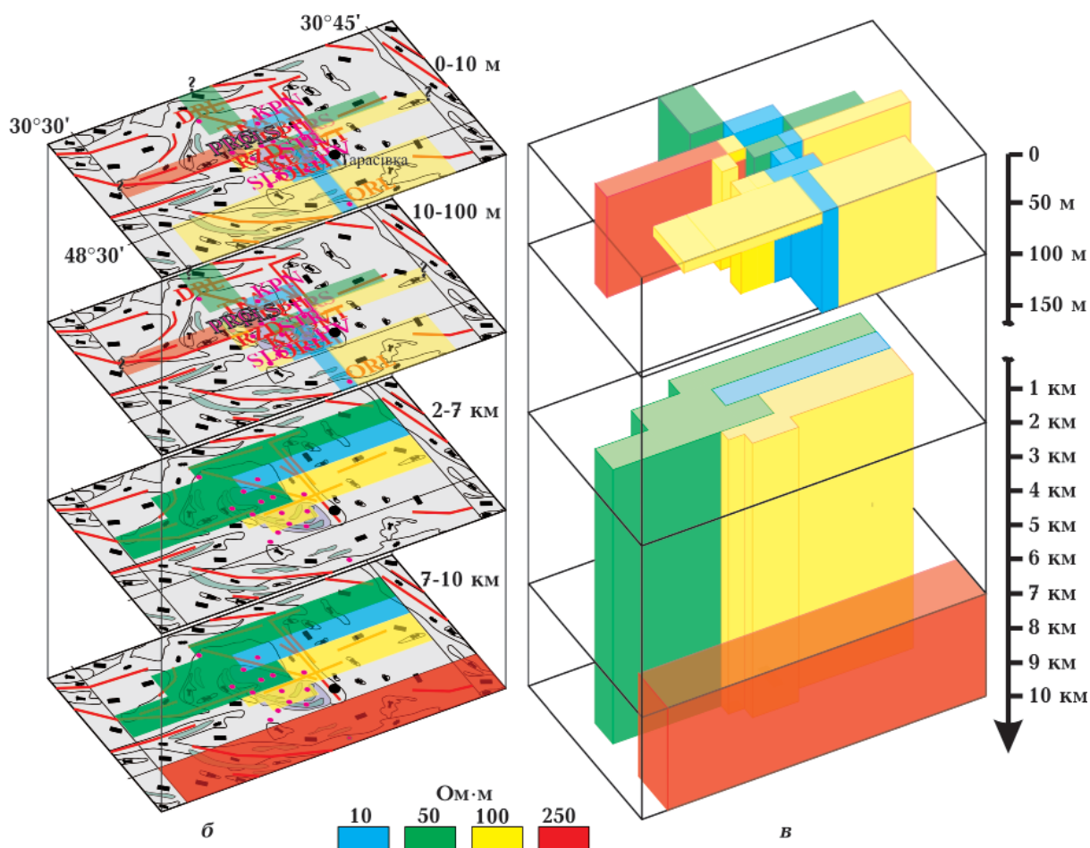
Рис. 7. Аномалії електропровідності планшета Тарасівської структури за результатами тривимірного моделювання електромагнітного поля: а — розподіл позитивного електричного опору (див. умовні позначення на рис. 4) Тарасівської структури за профілем А—В; б — на геолого-структурній карті поверхні кристалічного фундаменту ГШЗ, за даними [Гинтов и др., 2016], на глибинах 0—100 м та від 2 до 10 км; в — 3D геоелектрична модель.
