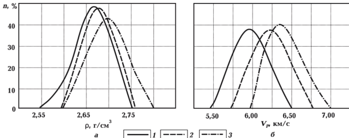
Рис. 2. Вариационные кривые распределения средних значений плотности (а) и скорости продольных волн (б) для гранитоидов: 1 — в атмосферных условиях ( V_{P0cp}=5,85 км/с; \rho_{0cp}=2,66 г/см 3 ); 2 — при воздействии на образцы высокого гидростатического давления 1 кбар ( V_{P1cp}=6,14 км/с; \rho_{1cp}=2,68 г/см 3 ); 3 — при воздействии на образцы высокого гидростатического давления 5 кбар ( V_{P5cp}=6,27 км/с; \rho_{5cp}=2,69 г/см 3 ).
