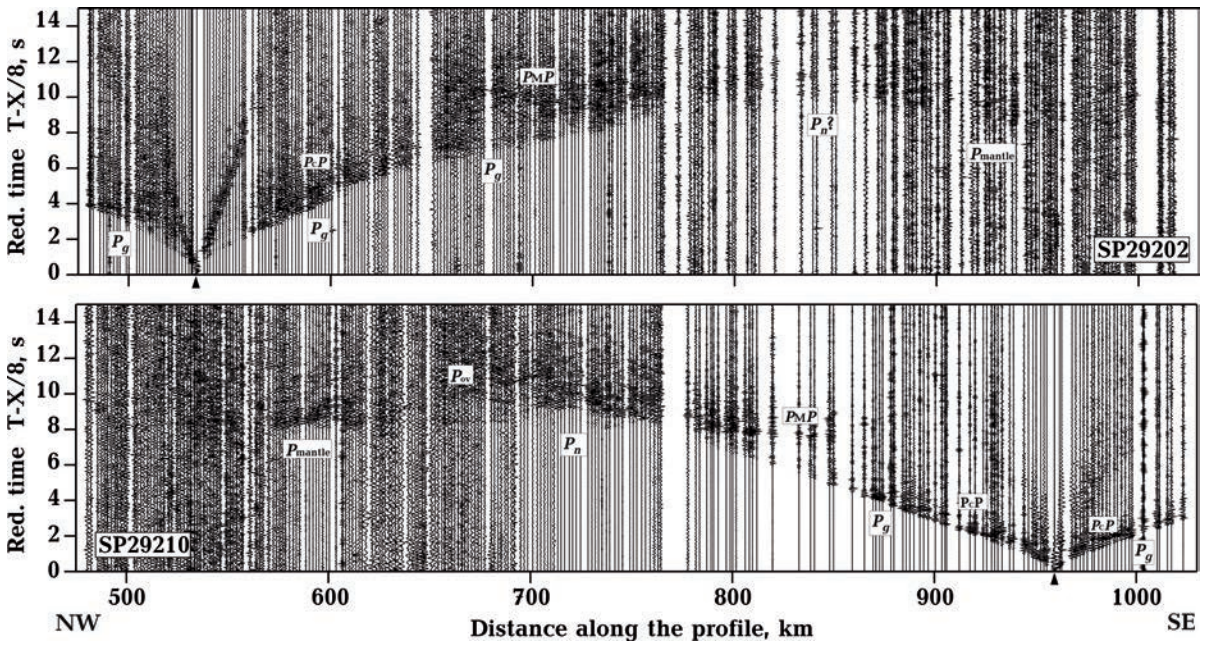
Рис. 3. Амплітудно-нормований сейсмічний розріз вертикальної складової поздовжніх P -хвиль пунктів вибуху SP29202 та SP29210. Швидкість редуції становить 8,0 км/с; P_g — заломлення у верхній та середній кристалічній корі; P_{ov} — закритична фаза хвилі в корі; P_c P — відбиття від межі в середній частині корі; P_M P — P -хвилі, відбиті від поверхні Мохо; P_n — заломлення у верхній мантії безпосередньо під поверхнею Мохо; P_{mantle} — фази P -хвиль у верхній мантії. Розташування пунктів вибуху показано на рис. 1.
