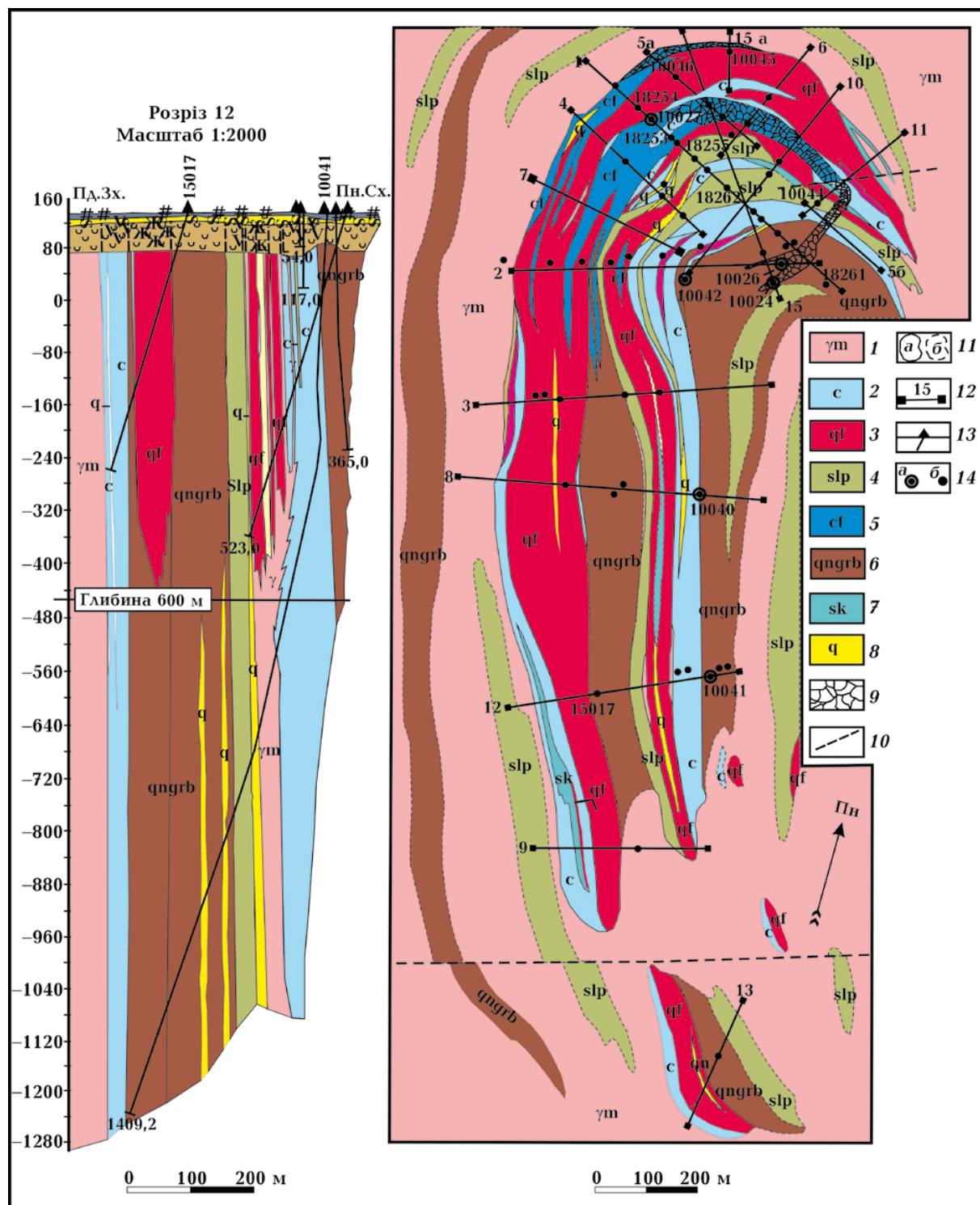
Рис. 7. Схематична геологічна карта м-бу 1:2000 Молдовського залізорудного родовища та геологічний розріз уздовж профілю 12, за матеріалами [Йонис і др., 1986]: 1 — граніти і мігматити; 2 — кальцифіри безрудні з олівіном, піроксеном і шпінеллю; 3 — кварцити залісті, переважно магнетит-феррогіперстенові і магнетит-дупіроксенові з гранатом; 4 — кристалосланці дупіроксен-плагіоклазові, що переходять в амфіболіти; 5 — кальцифіри рудні з магнетитом, олівіном, піроксеном, шпінеллю, іноді з кліногумітом; 6 — гнейси гранат-біотитові і біотитові з силманітом і кордієритом, гнейси графітові і піроксенові; 7 — скарни безрудні піроксенові і гранат-піроксенові; 8 — кварцити безрудні гіперстенові, гранат-гіперстенові і біотит-гранат-гіперстенові; 9 — зони дроблення і брекчіювання; 10 — розривні порушення; 11 — геологічні
