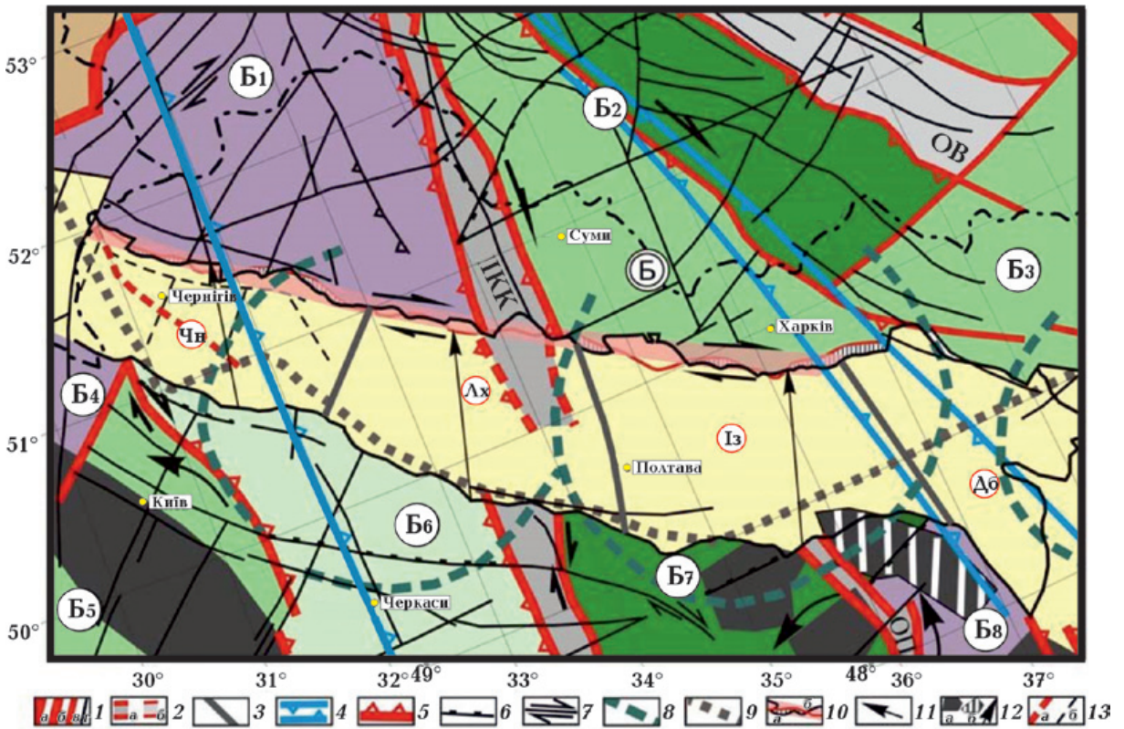
Рис. 14. Фрагмент Схеми тектонічного районування кристалічного фундаменту Сарматії, за [Старостенко и др., 2017] (світло-зеленим показано грабен ДДЗ): 1 — розломи (а — міжгеоблокові, б — міжмегаблокові, в — міжблокові, г — інші); 2 — шовні зони першого (а) та другого (б) рангу; 3 — міжсегментні розломи ДДЗ; 4 — трансрегіональні тектонічні шви; 5–8 — кінематичні типи розломів (5 — насуви, 6 — скиди, 7 — зсуви, 8 — кільцеві структури, виділені за аерокосмічними даними); 9 — північна межа поширення високошвидкісного прошарку в перехідній зоні верхньої мантії [Цветкова, Бугаєнко, 2012]; 10 — положення суміщених північного (чорний) і південного (червоний) крайових розломів грабену ДДЗ та передбачуване положення дорифтової шовної зони (рожева смуга); перекриття (а) та «зіяння» (б) при суміщенні; 11 — напрямком переміщення південного крайового розлому для оптимального поєднання з північним; 12 — давні ядра консолідації кори (а), перероблені з направленням їх обертання під час формування рифту, за [Чекунів, Пашкевич, 1989] (б); 13 — положення розломів УЩ після поєднання крайових розломів ДДЗ. Літери у великих кружках — блоки першого рангу ВМ і мегаблоки УЩ: Б1 — Брянський, Б2 — Курський, Б3 — Россошанський, Б4 — Волинський, Б5 — Росинський, Б6 — Інгульський, Б7 — Середньопридніпровський, Б8 — Приазовський. Шовні зони: ІКК — Інгулецько-Криворізько-Крупецька та ОП — Оріхів-Павлоградська І-го рангу, ОВ — Олексіївсько-Воронезька ІІ-го рангу. Літери у малих кружках — блоки ДДЗ: Чн — Чернігівський, Лх — Лохвицький, Із — Ізюмський, Дб — Донбаський.
