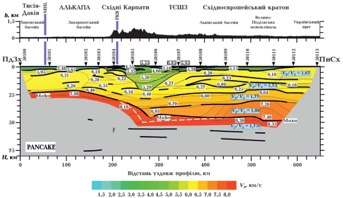
Рис. 10. Двовимірний модель швидкості P -хвиль в корі та верхній мантії, отримана прямим моделюванням трасування променів за допомогою пакету SEIS83 [Červený, Pšenčík, 1984] уздовж профілю DOBRE-3 (PANCAKE), за [Starostenko et al., 2013a]. Товсті чорні лінії — великі розриви швидкості (інтерфейси першого порядку). Товсті переривчасті лінії — частини розривів першого порядку, обмежені відбитими та/або заломленими надходженнями P -хвиль. Тонкі лінії — ізолінії швидкості зі значеннями в км/с, показаними в білих прямокутниках. Стрілки показують положення пунктів вибуху, сині стрілки — перетини з іншими профілями. Співвідношення вертикального і горизонтального масштабів становить \sim 2,4:1 . Для СЕК показано модель розподілу співвідношення V_P/V_S . Біла пунктирна лінія — глибина межі поділу Мохо, якщо використовувати швидкість \sim 7,2 км/с замість 6,9 км/с у нижній частині кори. МНЛ — Середньоугорська лінія, РКВ — Пеннінський келіповий пояс.
