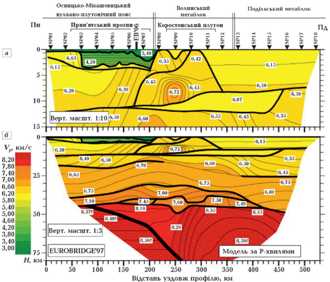
Рис. 9. Двовимірний модель швидкості P -хвилі за профілем EUROBRIDGE'97 [Thybo et al., 2003]: a — деталі верхньої кори; б — повна літосферна модель. Товсті чорні лінії — основні швидкісні межі. Відбивач у мантії обмежений лише відбиттями, тому швидкість під ним невідома. Тонкі лінії — ізолінії швидкості зі значеннями (км/с), показаними в білих прямокутниках. Стрілки показують положення пунктів вибуху.
