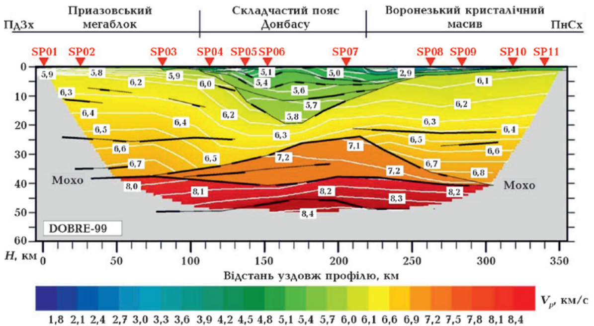
Рис. 13. Швидкісна модель позовжніх хвиль по профілю DOBRE-99 через складчастий пояс Донбасу, Приазовський мегаблок і Воронежський масив, за [Grad et al., 2003]. Вертикальна шкала — глибина під поверхнею в км. Ізолінії швидкості проведені з інтервалом 0,1 км/с (білі прямокутники). Товсті лінії — положення якісних відбивних границь.
