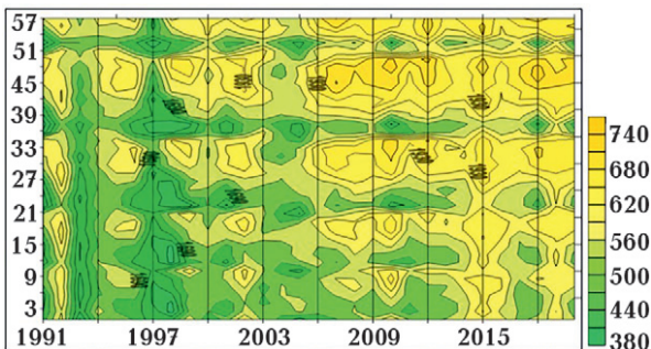
Рис. 3. Зміни сумарної сонячної радіації ( \text{МДж/м}^2 ) на території України протягом літнього сезону упродовж 1991—2020 рр.
