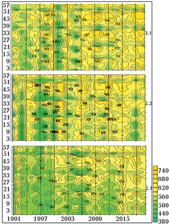
Рис. 2. Зміни сумарної сонячної радіації ( \text{МДж/м}^2 ) на території України упродовж 1991—2020 рр.: а — у червні, б — у липні, в — у серпні.
