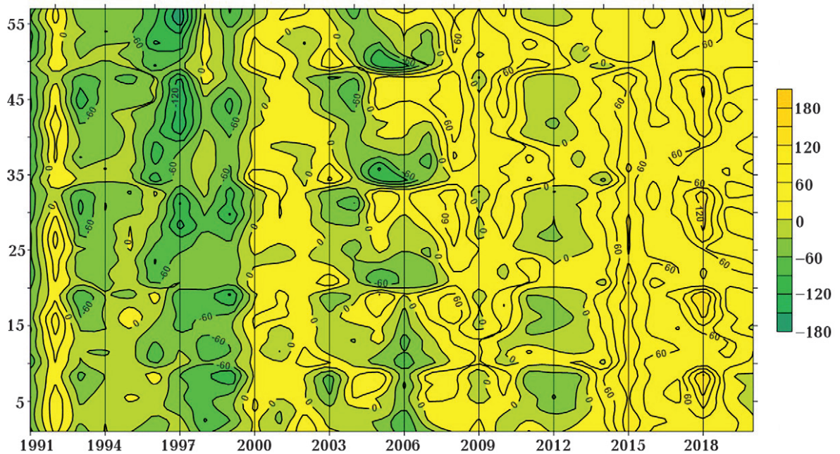
Рис. 6. Відхилення прямої сонячної радіації ( \text{МДж/м}^2 ) від середнього значення у вузлах регулярної сітки над територією України в серпні 1991—2020 рр.
