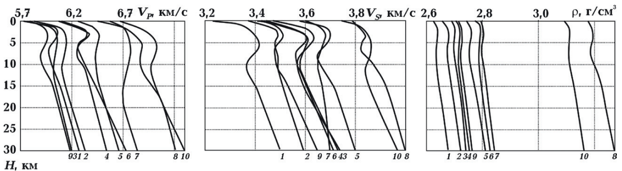
Рис. 4. Зміни швидкостей V_P , V_S і \rho за термодинамічних умов на різній глибині: 1 — рівномірнозернисті граніти, 2 — порфіроподібні граніти, 3 — новотуркські граніти та граніти рапаківі, 4 — плагіограніти, 5 — чарнокітоїди, 6 — породи середнього складу, 7 — породи основного складу, 8 — піроксеніти, 9 — гнейси біотитові, 10 — гнейси амфібол-піроксенового складу.
