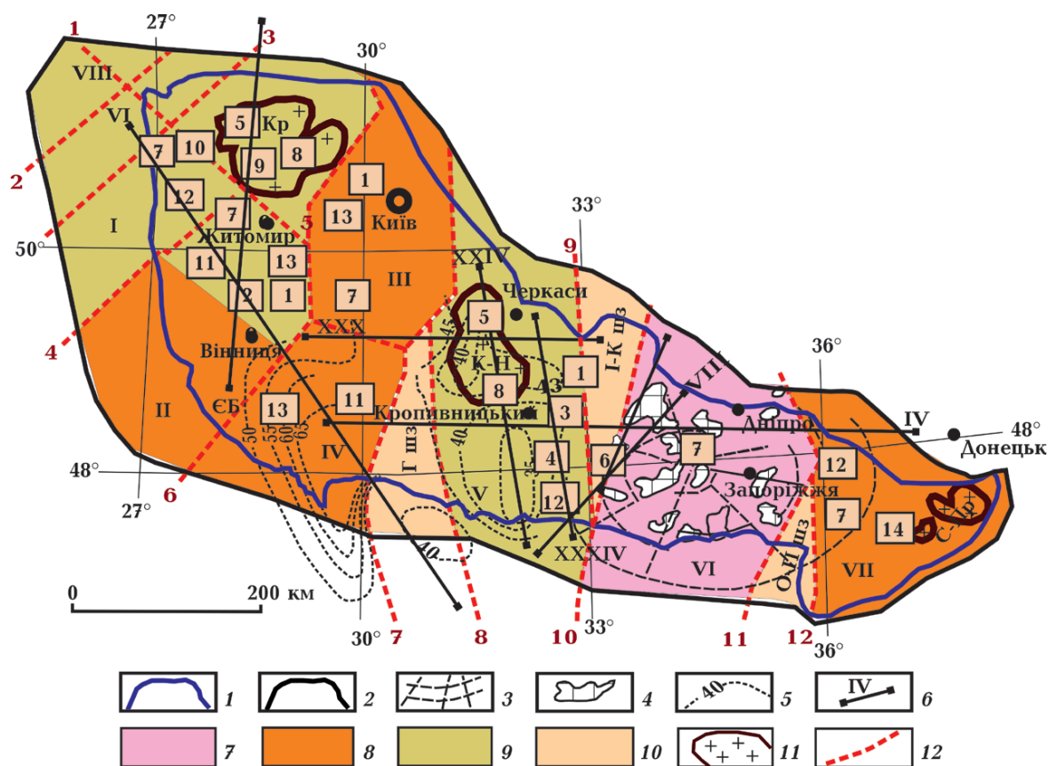
Рис. 2. Схема структурно-тектонічного районування Українського щита (за [Кировоградський ..., 2013; Гінтов та ін., 2018]) і розміщення місць відбору зразків досліджених порід: 1 — контур відслоненої частини щита; 2 — контур схилів щита, в межах яких простежуються складчасті та розривні структури докембрійського фундаменту за геофізичними даними; 3 — Придніпровське палеосклепіння; 4 — зеленокам'яні синклінорії; 5 — ізоглибини поділу Мохо, км; 6 — сейсмічні геотрансекти; комплекси порід: 7 — архейські, 8 — архейські, перероблені в протерозой, 9 — палеопротерозойські; 10 — шовні зони (Гшз — Голованівська, І-Кшз — Інгuleцько-Криворізька, О-Пшз — Оріхів-Павлоградська); 11 — масиви (Кр — Коростенський, К-Н — Корсунь-Новомиргородський, С-Пр — Східноприазовський); 12 — міжмегаблокові розломи (1 — Центральний, 2 — Луцький, 3 — Суццано-Пержанський, 4 — Тетерівський, 5 — Брусилівський, 6 — Немирівський, 7 — Тальнівський, 8 — Первомайський, 9 — Західноінгулецький, 10 — Криворізько-Кременчуцький, 11 — Оріхів-Павлоградський, 12 — Азово-Павлоградський). Мегаблоки (римські цифри): I — Волинський; II — Подільський; III — Росинський; IV — Бузький; V — Інгuleцький; VI — Середньопридніпровський; VII — Приазовський; VIII — Волино-Подільський вулканоплутонічний пояс. Місця відбору зразків порід (цифри в квадратах): 1—5 — граніти (1 — рівномірнозернисті, 2 — гранат-біотитові чудново-бердичівські, 3 — порфіроподібні біотитові, 4 — порфіроподібні трахітоїдні новоукраїнські, 5 — рапаківи); 6 — плагіограніти; 7 — діорити, гранодіорити; 8 — лабрадорити; 9 — габро; 10 — піроксеніти; 11 — чарнокітоїди; 12 — гнейси біотитові; 13 — гнейси піроксенові, амфіболові; 14 — породи приазовського лужного комплексу.
