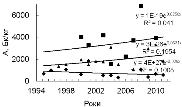
Рис. 5. Часові тенденції змін вмісту ^{137}\text{Cs} у білих (♦) і польських (■) грибах та лисичках (Δ) з ШНПП.
