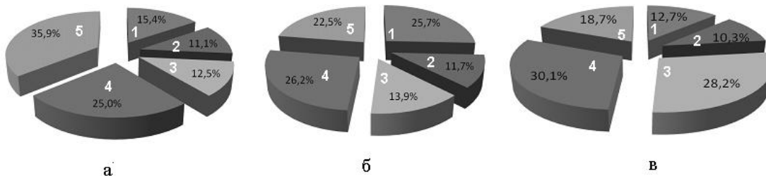
Рис. 4. Розподіл питомої активності ^{137}\text{Cs} у частинах рослин (а – брусниця; б – лохина; в – чорниця) з Шацького національного природного парку: 1 – коріння; 2 – старі пагони; 3 – цьогорічні пагони; 4 – листя; 5 – ягоди.
