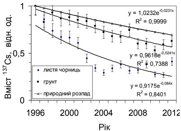
Рис. 2. Динаміка природного розпаду та зміни вмісту ^{137}\text{Cs} у ґрунті й листі чорниць у 1996-2012 рр.
