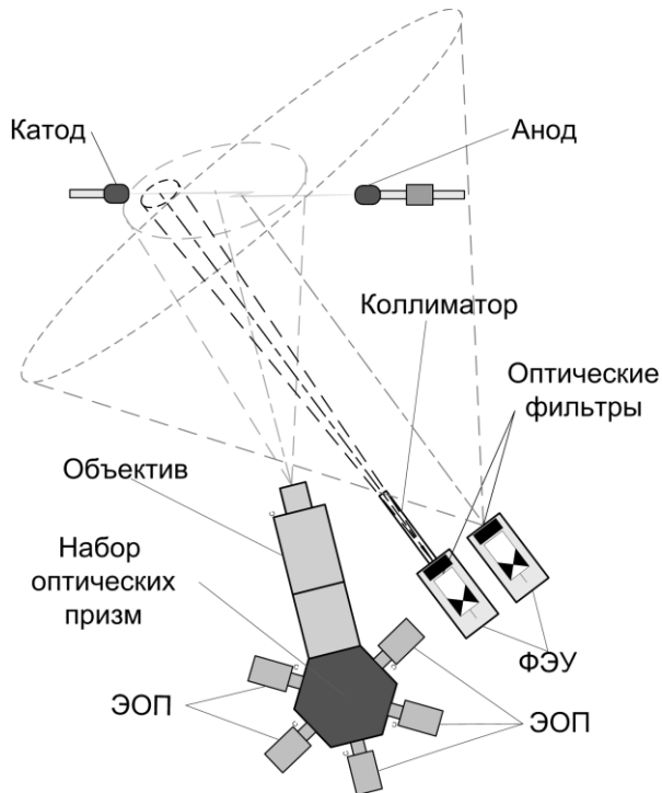
Рис. 5. Схема расположения диагностик в проведенных экспериментах.
