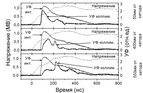
Рис. 7. Результаты проведенных экспериментов по обнаружению области генерации УФ излучения на начальных стадиях развития протяженного высоковольтного искрового разряда.
