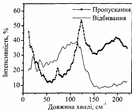
Рис. 1. ІЧ спектри пропускання і відбивання кристала 4H\text{-CdI}_2 .
